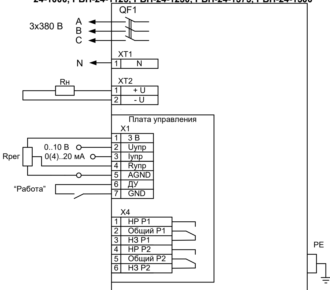
Рисунок А3 Схема подключения РБП-24-375, РБП-24-500, РБП-24-625, РБП-24-750, РБП-24-875, РБП-24-1000, РБП-24-1125, РБП-24-1250, РБП-24-1375, РБП-24-1500, питание – трехфазное с нулевым проводом
