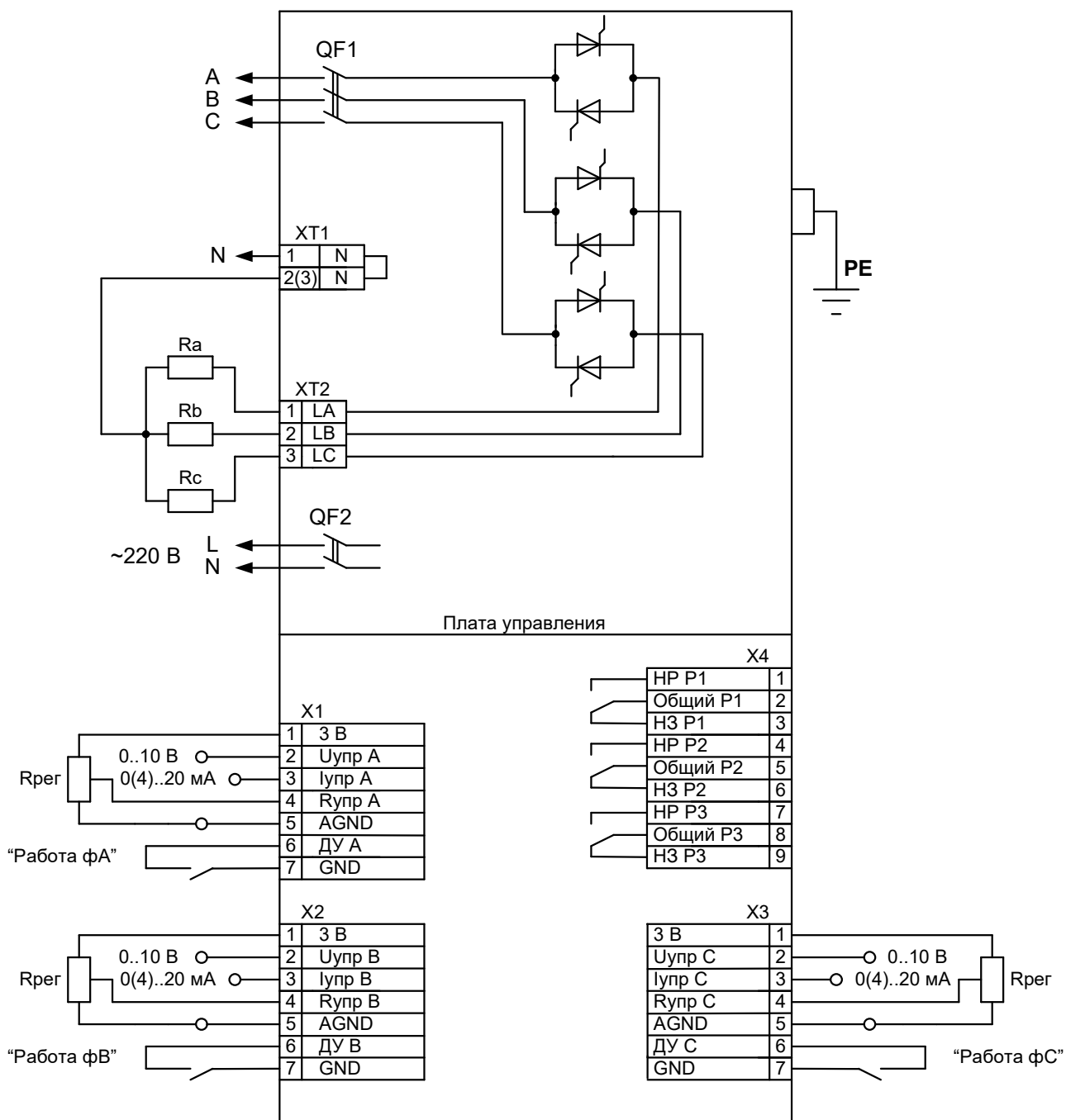
Рисунок А1 Схема подключения нагрузки – “звезда” с рабочей нейтралью
