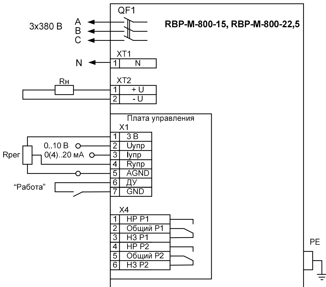
Рисунок А2 Схема подключения RBP-M-800-15, RBP-M-800-22,5, питание – трехфазное с нулевым проводом
