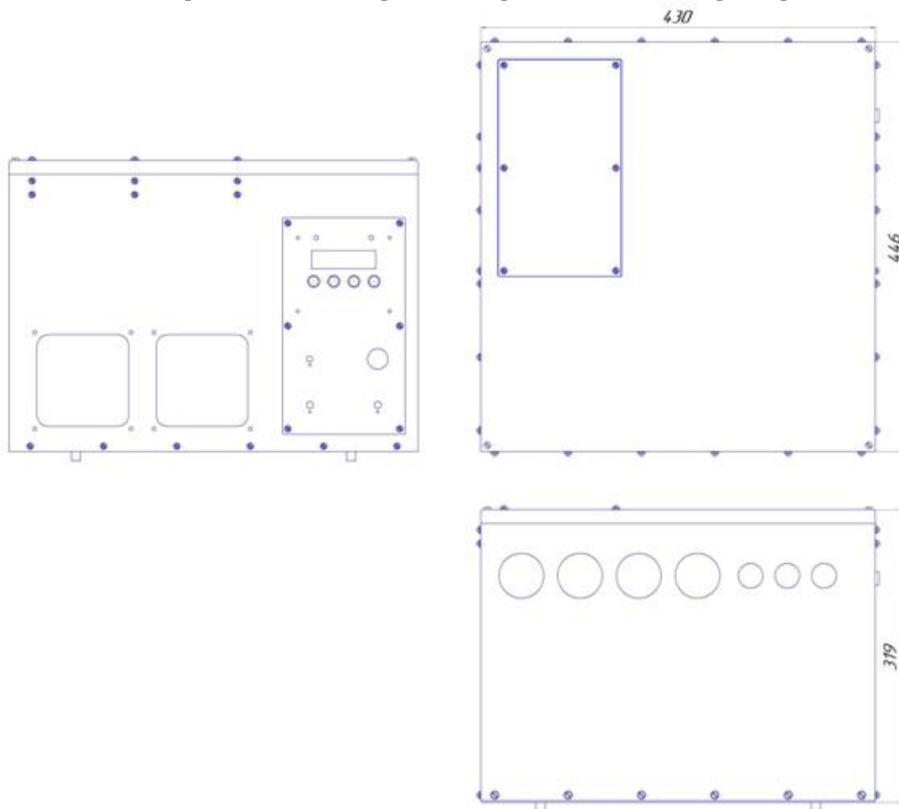
Рисунок Б1 Настольный вариант использования RBP-M-800-7,5
