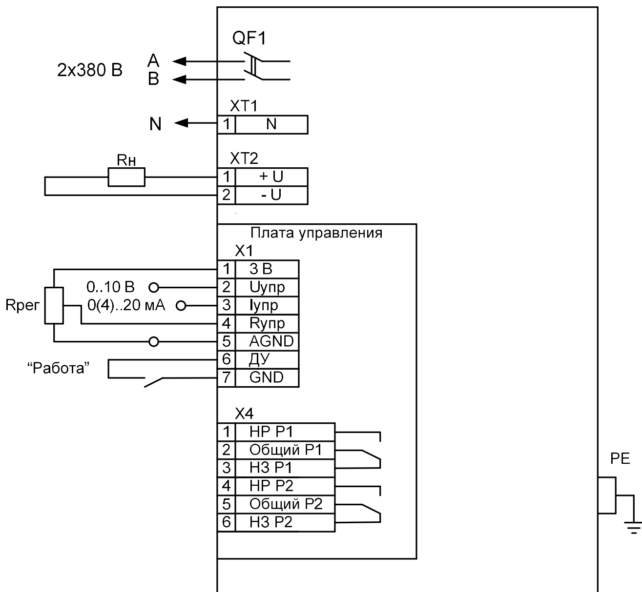
Рисунок А1 Схема подключения RBP-M-800-7,5, питание – двухфазное с нулевым проводом
