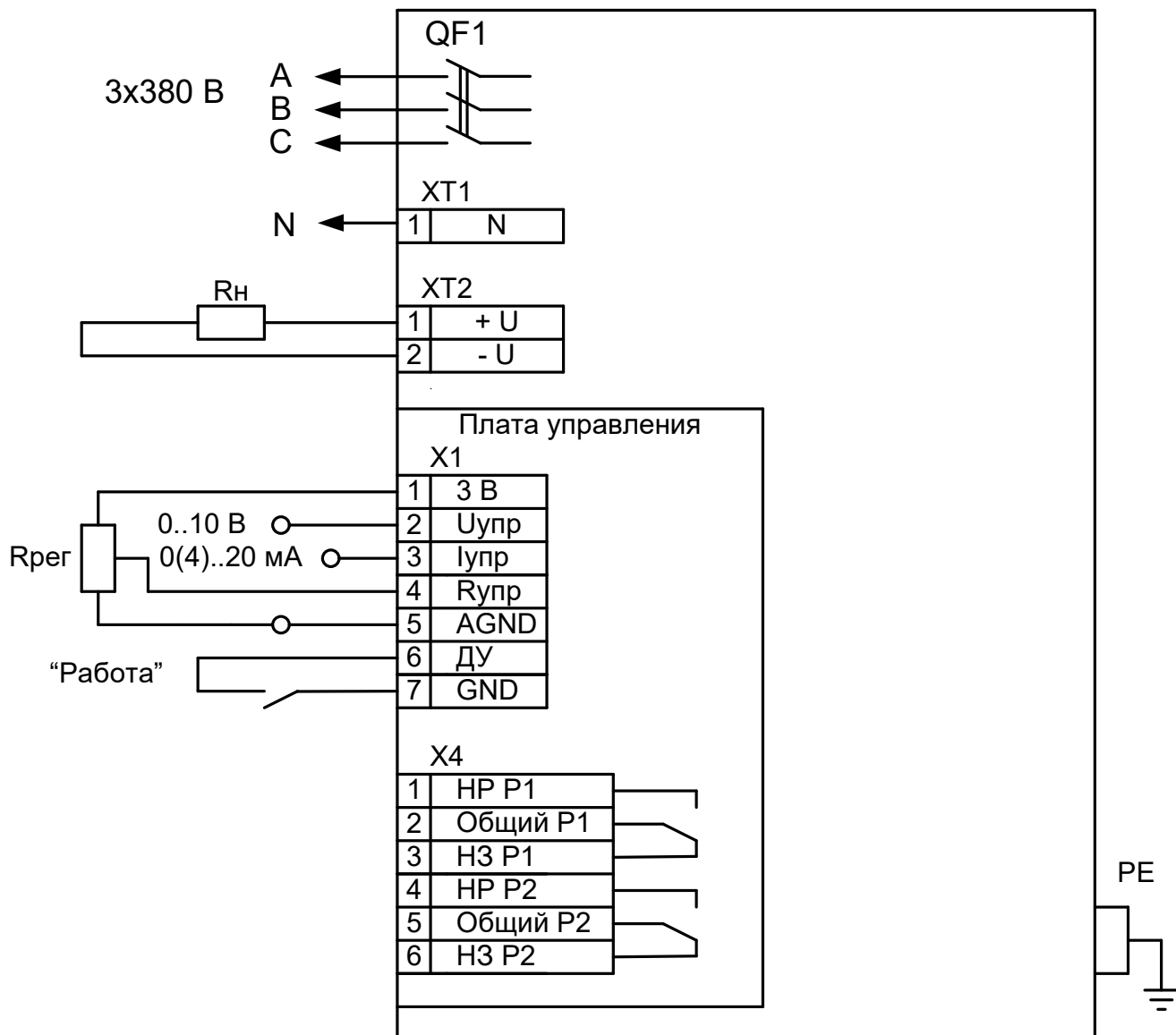
Рисунок А3 Схема подключения РБП-384-62, питание – трехфазное с нулевым проводом
