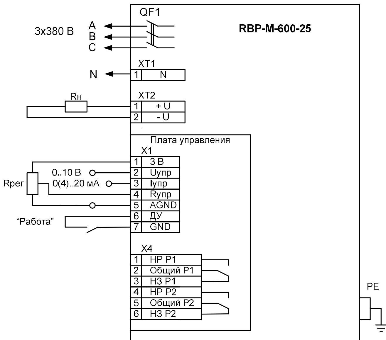
Рисунок А1 Схема подключения RBP-M-600-25, питание – трехфазное с нулевым проводом
