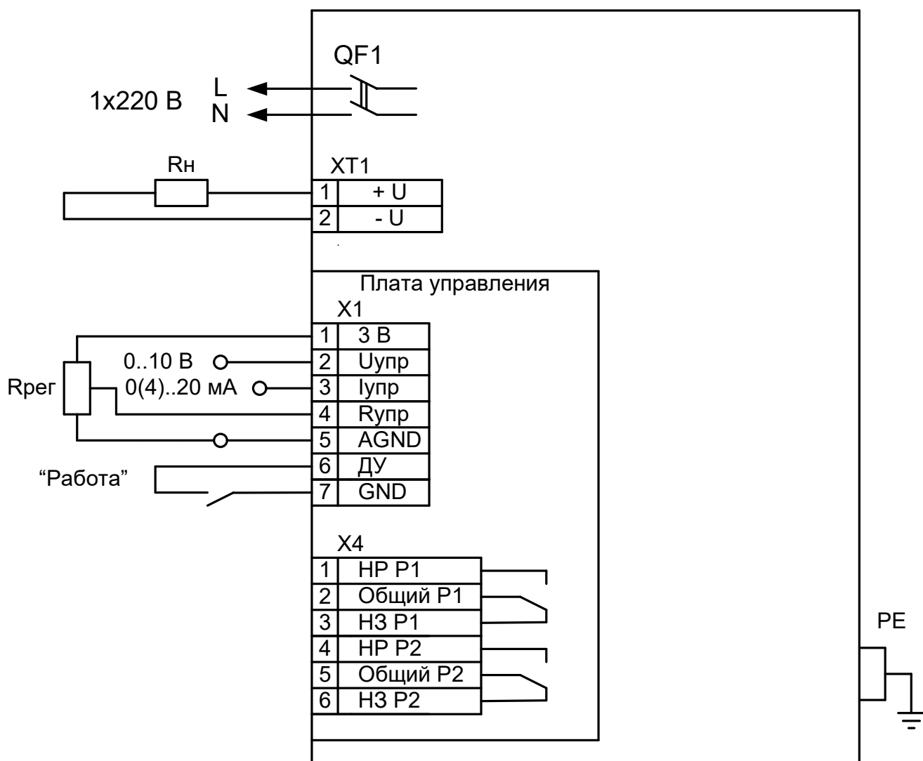
Рисунок А1 Схема подключения РБП-М-400-7,5, питание - однофазное
