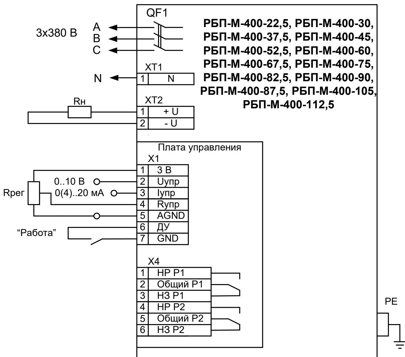
Рисунок А3 Схема подключения РБП-М-400-22,5 РБП-М-400-30, РБП-М-400-37,5, РБП-М-400-45, РБП-М-400-52,5, РБП-М-400-60, РБП-М-400-67,5, РБП-М-400-75, РБП-М-400-82,5, РБП-М-400-90, РБП-М-400-97,5, РБП-М-400-105, РБП-М-400-112,5, питание – трехфазное с нулевым проводом
