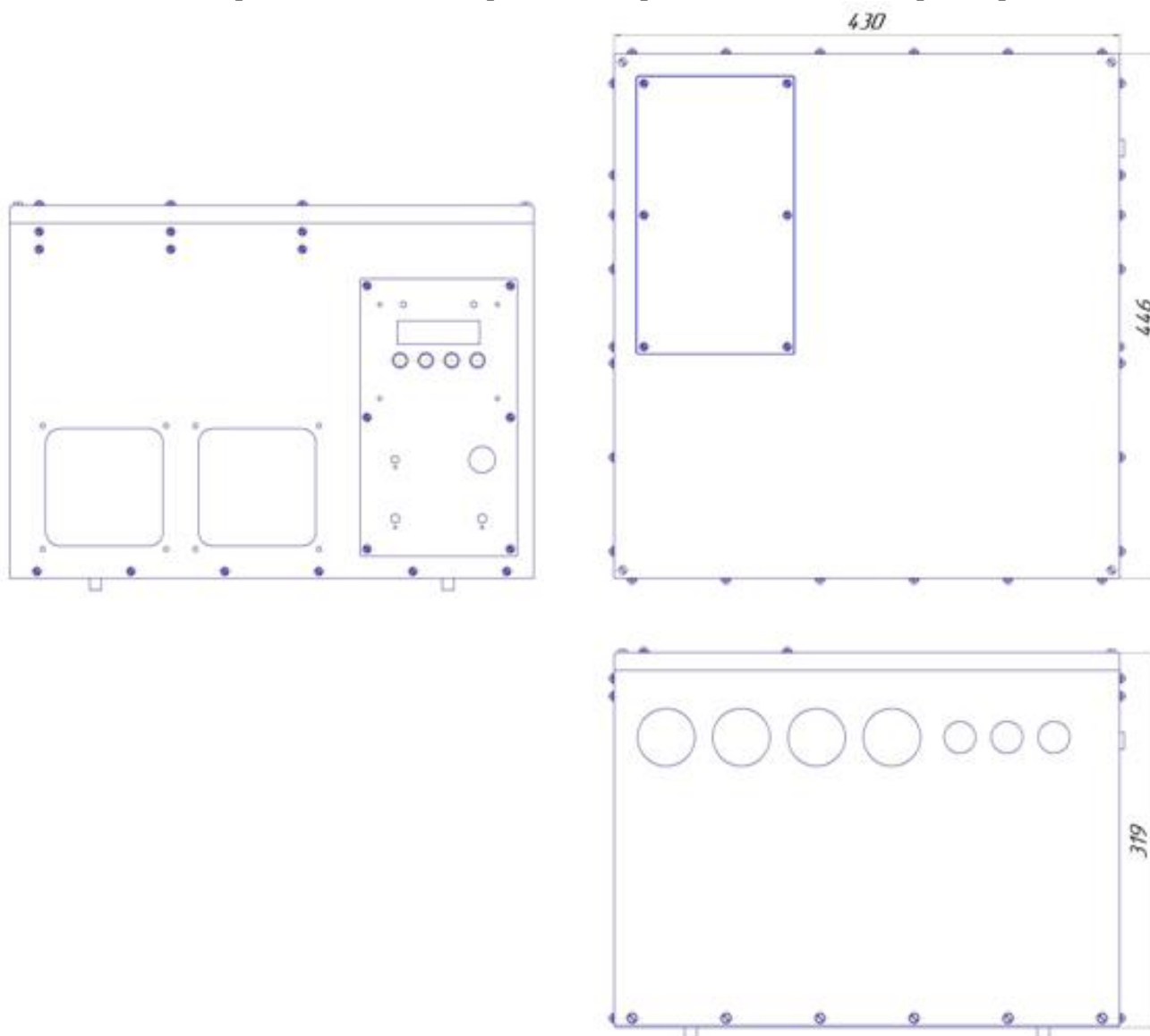
Рисунок Б1 Настольный вариант использования RBP-R-M-360-25
