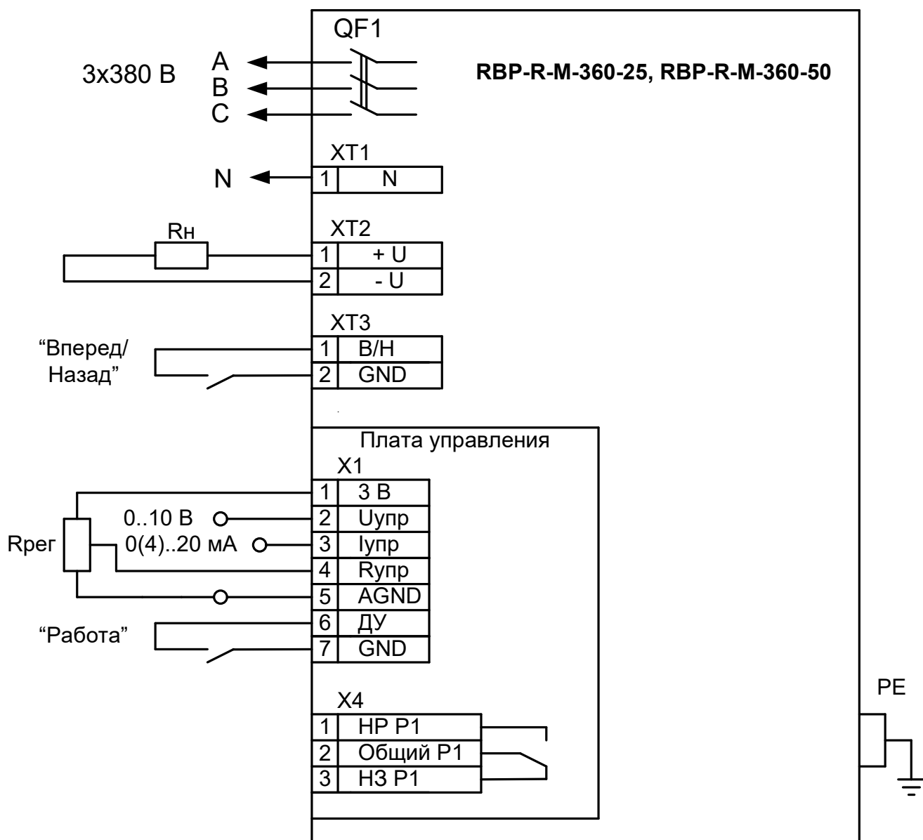
Рисунок А2 Схема подключения RBP-R-M-360-25, RBP-R-M-360-50, питание – трехфазное с нулевым проводом
