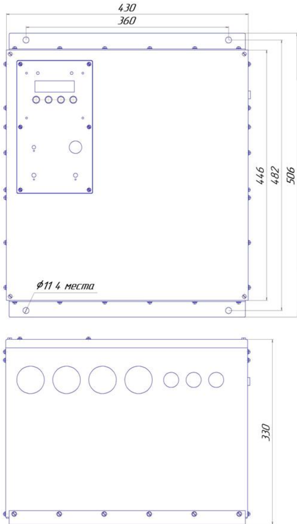
Рисунок Б3 Навесной вариант использования RBP-R-M-360-25. Крепежные уголки – сверху и снизу.
