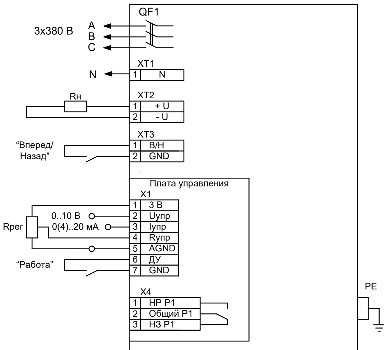
Рисунок А1 Схема подключения РБП-Р-480-62, питание – трехфазное с нулевым проводом
