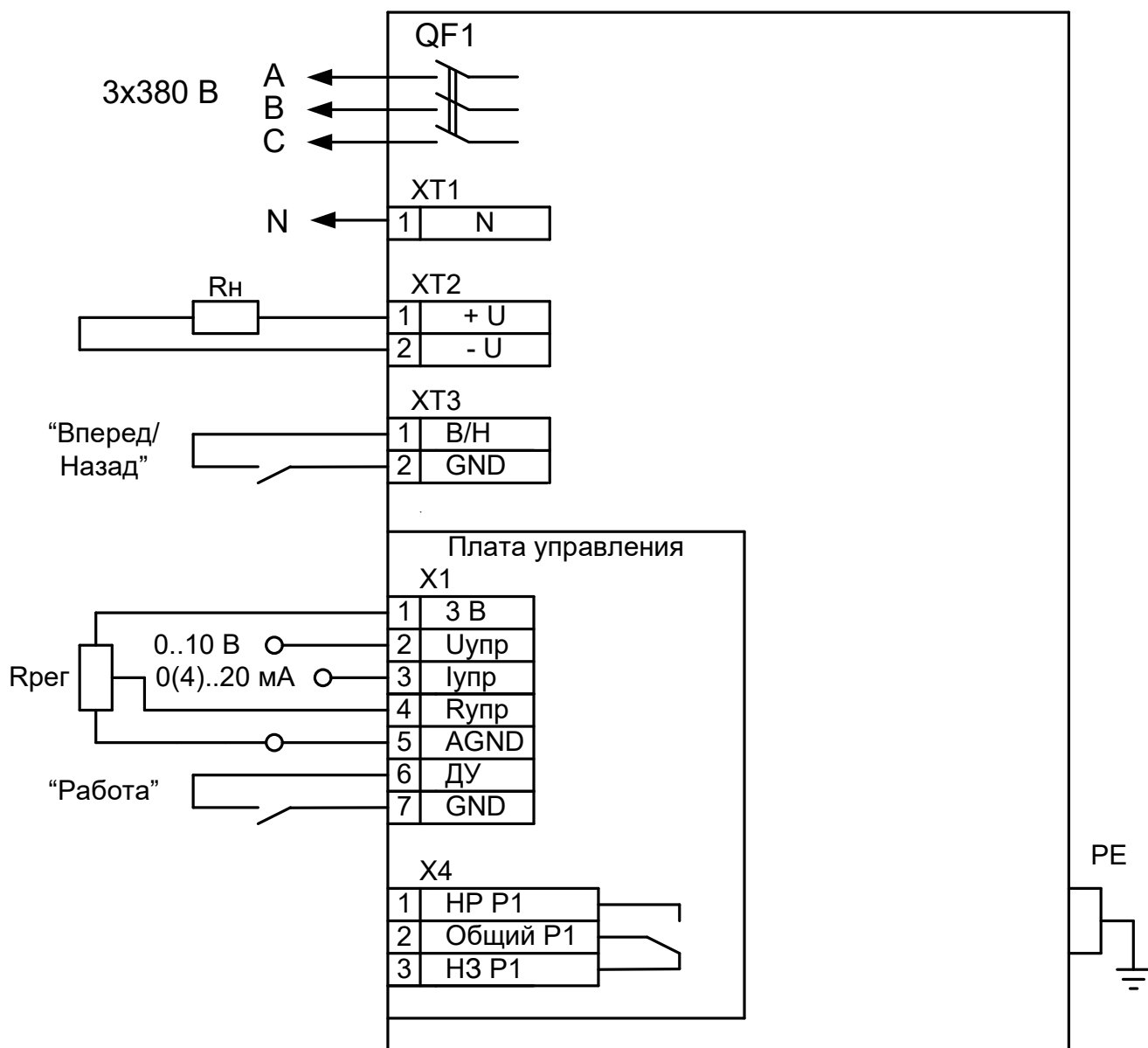
Рисунок А1 Схема подключения RBP-R-36, питание – трехфазное с нулевым проводом
