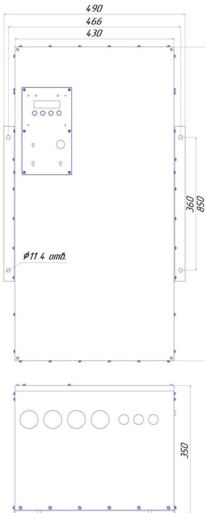
Рисунок Б5 Навесной вариант использования RBP-R-36-400. Крепежные уголки слева и справа
