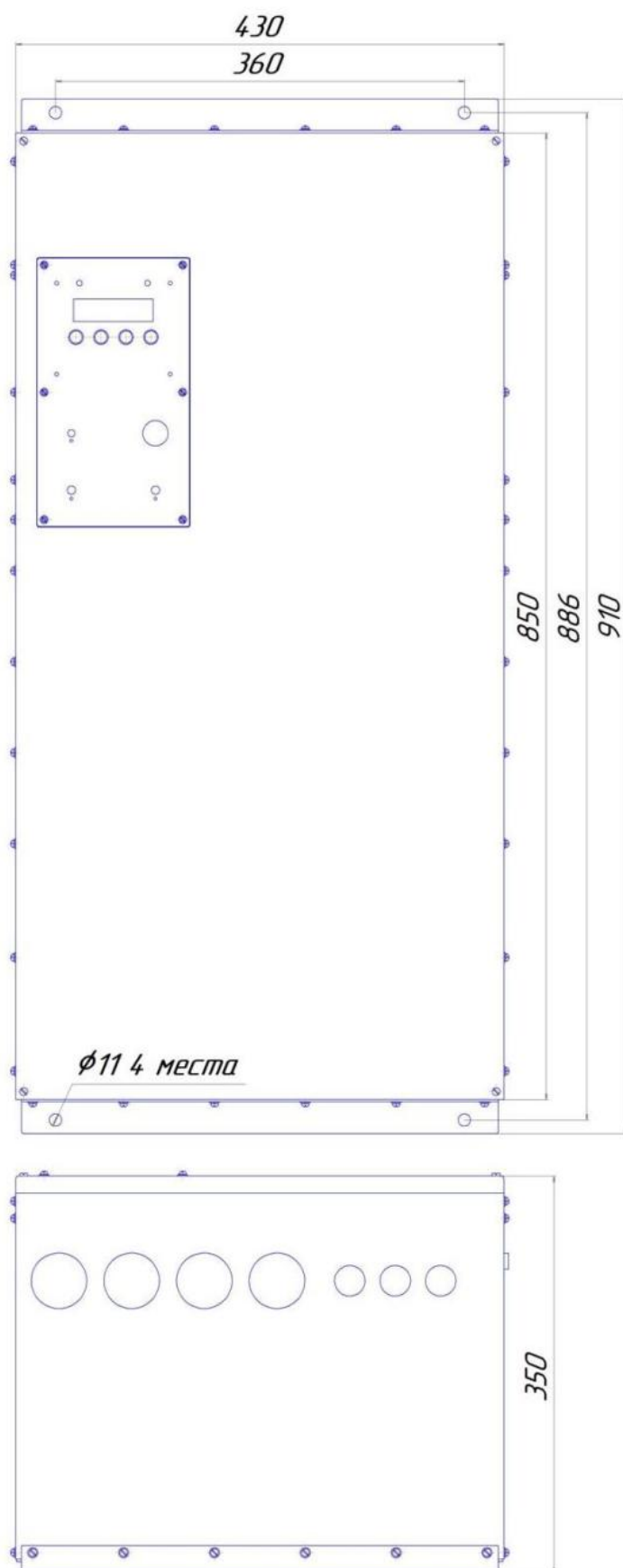
Рисунок Б6 Навесной вариант использования RBP-R-36-400. Крепежные уголки – сверху и снизу.
