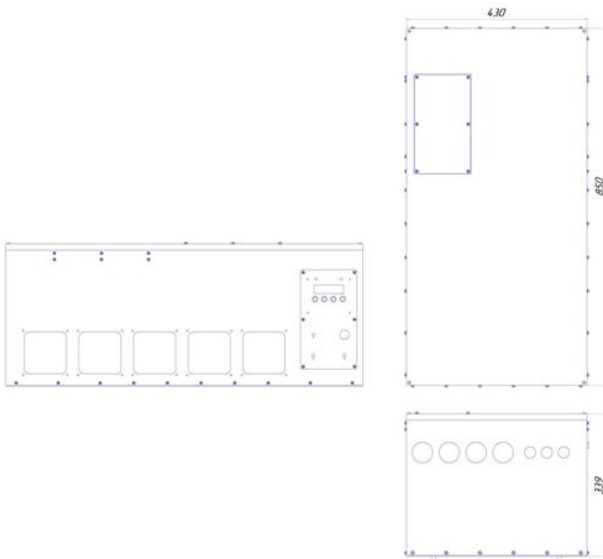
Рисунок Б4 Настольный вариант использования RBP-R-36-400
