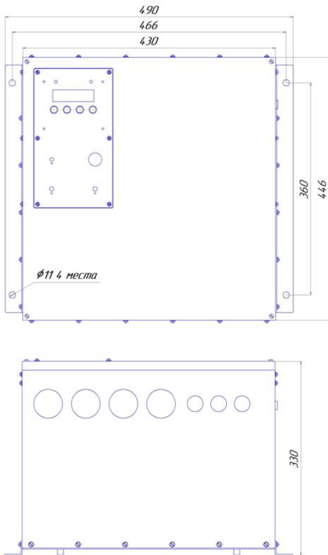
Рисунок Б2 Навесной вариант использования RBP-R-144-62. Крепежные уголки – слева и справа.
