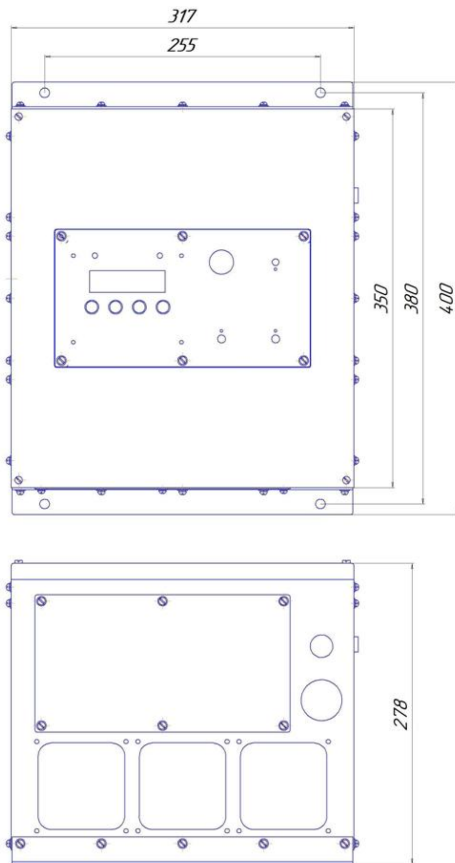
Рисунок Б3 Навесной вариант использования RBP-24-125. Крепежные уголки – сверху и снизу.
