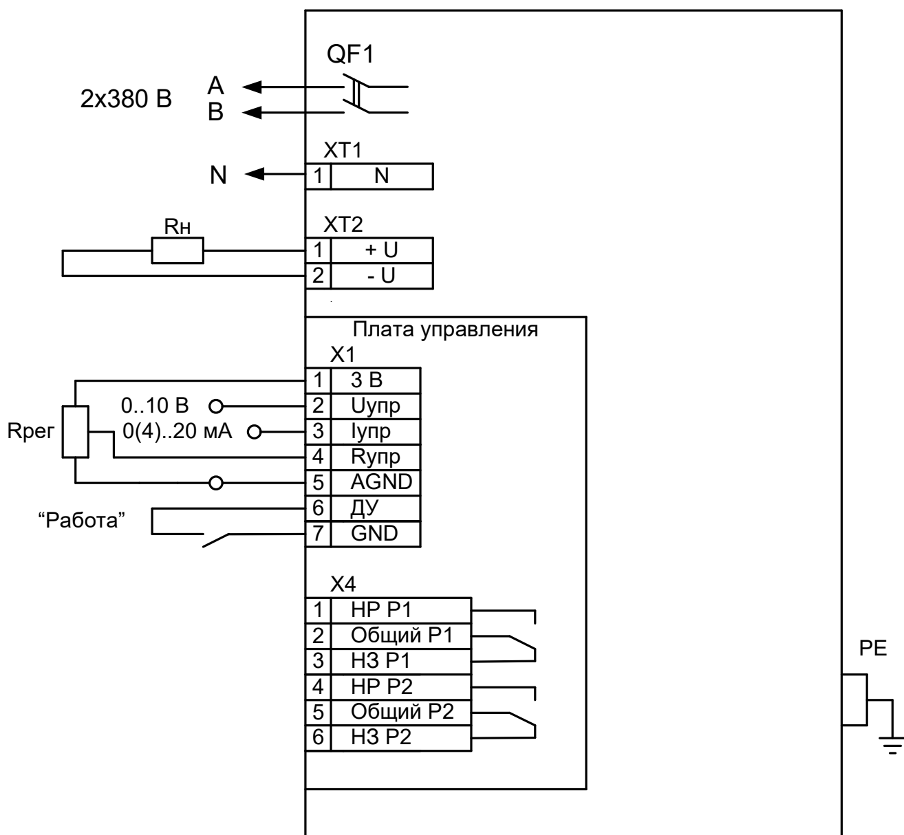
Рисунок А2 Схема подключения RBP-24-250, питание – двухфазное с нулевым проводом
