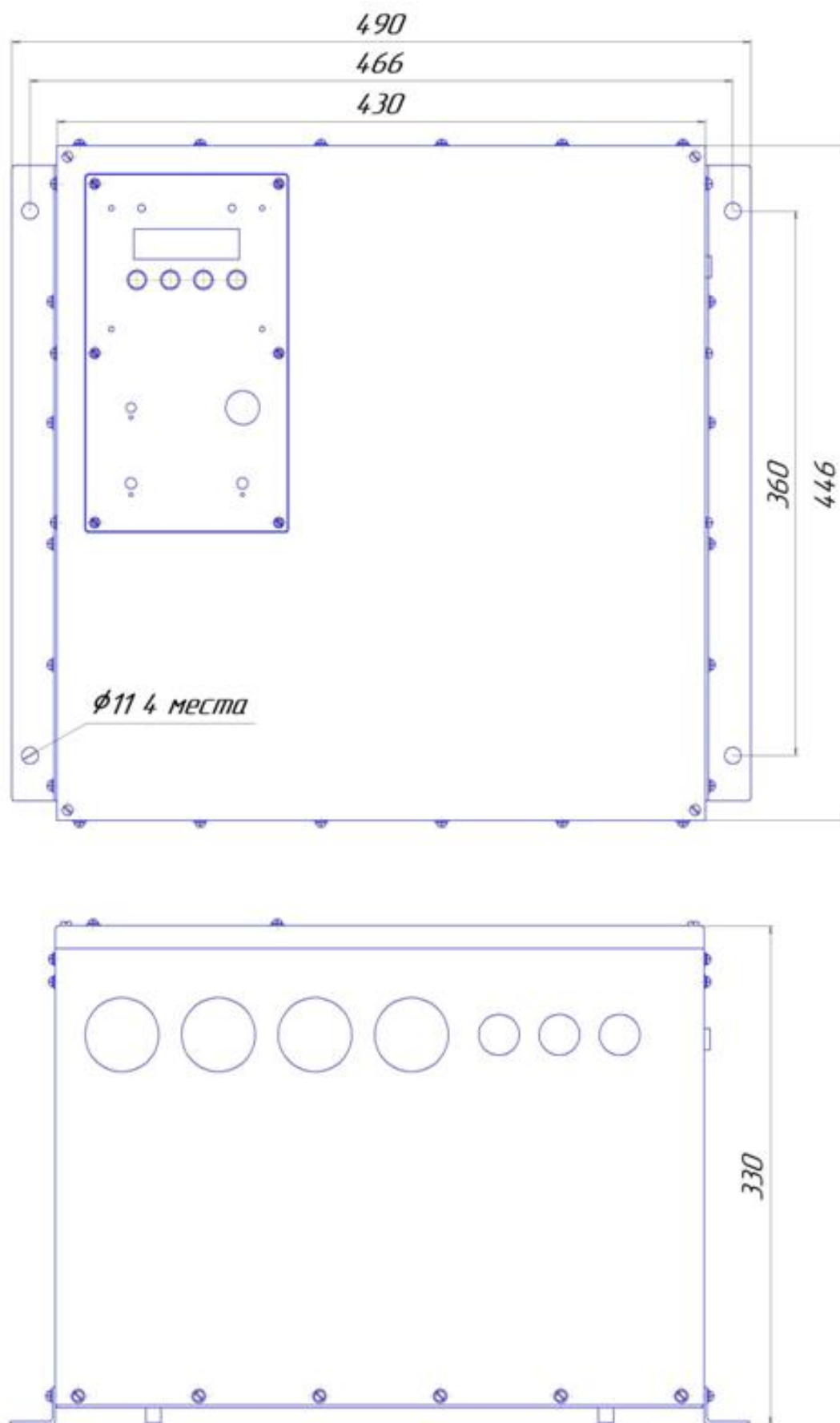
Рисунок Б5 Навесной вариант использования RBP-24-250, RBP-24-375. Крепежные уголки – слева и справа.
