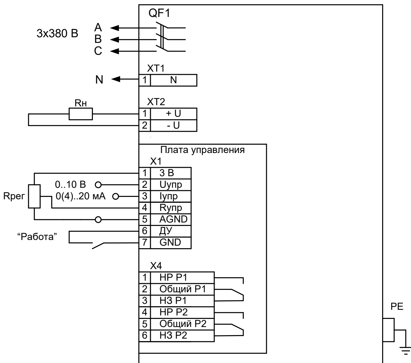
Рисунок А3 Схема подключения RBP-24-375, RBP-24-500, RBP-24-625, RBP-24-750, питание – трехфазное с нулевым проводом
