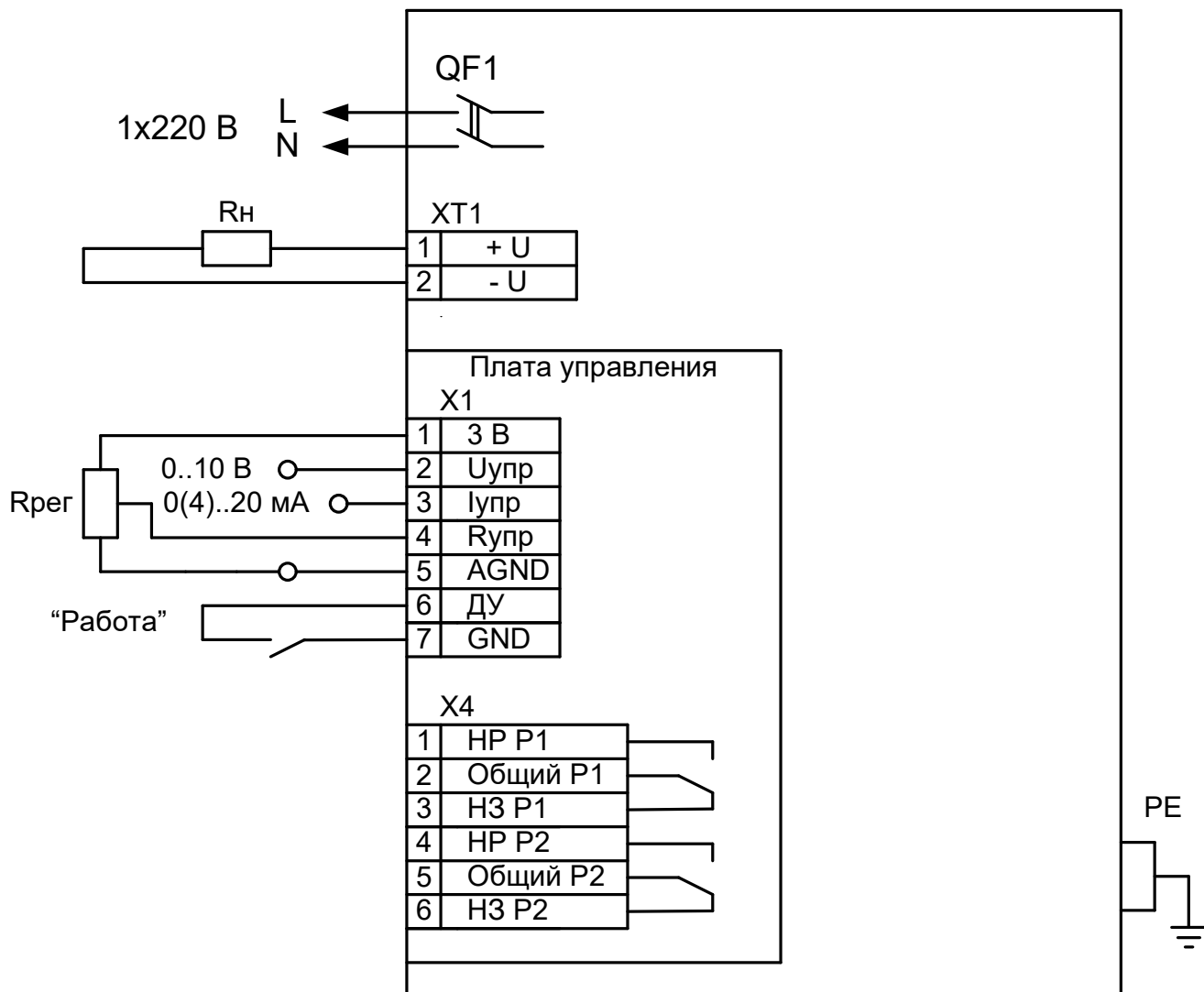
Рисунок А1 Схема подключения RBP-24-125
