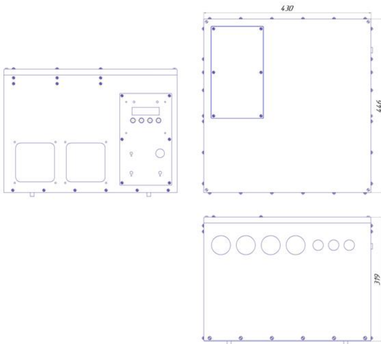
Рисунок Б1 Настольный вариант использования RBP-R-72-125
