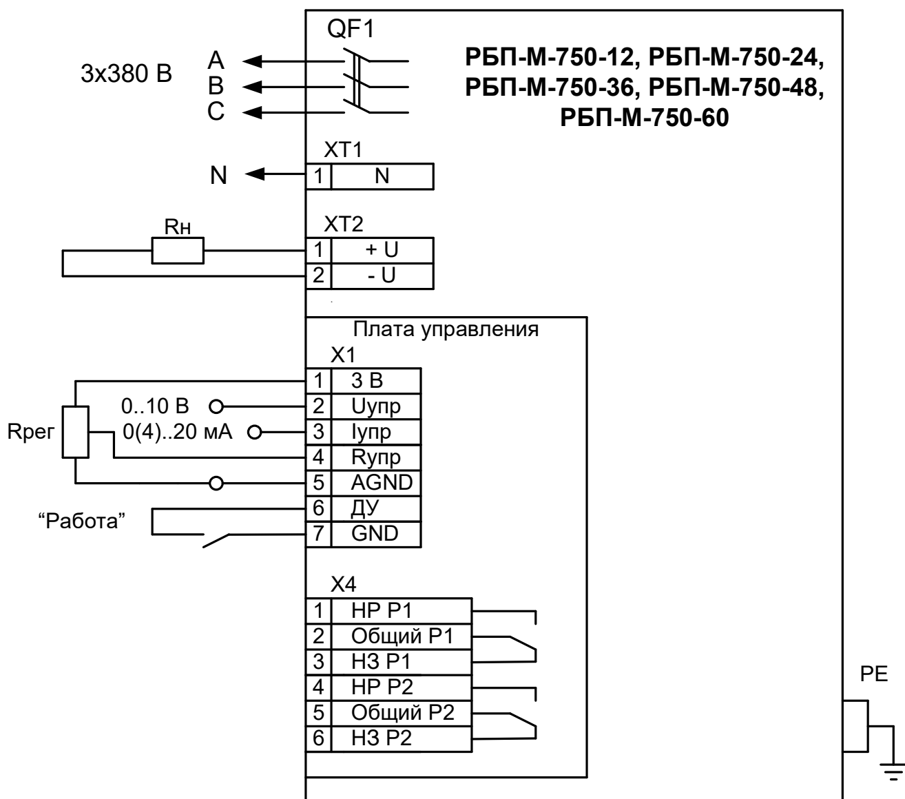
Рисунок А1 Схема подключения РБП-М-750-12, РБП-М-750-24, РБП-М-750-36, РБП-М-750-48, РБП-М-750-60, питание – трехфазное с нулевым проводом
