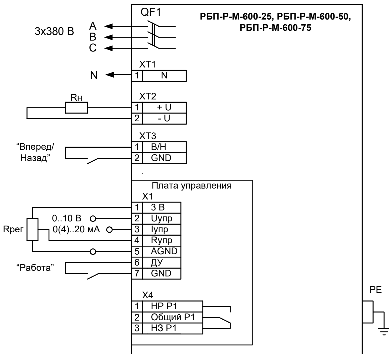
Рисунок А1 Схема подключения РБП-Р-М-600-25, РБП-Р-М-600-50, РБП-Р-М-600-75, питание – трехфазное с нулевым проводом
