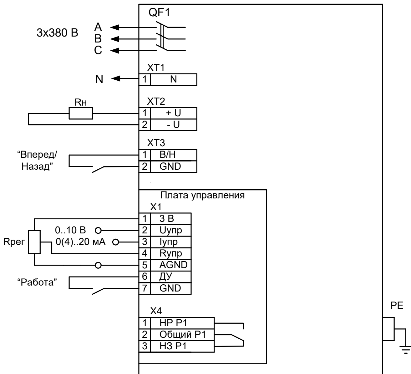
Рисунок А1 Схема подключения RBP-R-192-62, питание – трехфазное с нулевым проводом
