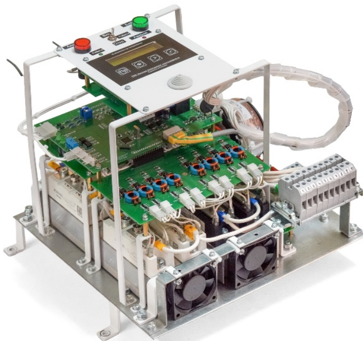
Рисунок 3.4 Тиристорный блок
