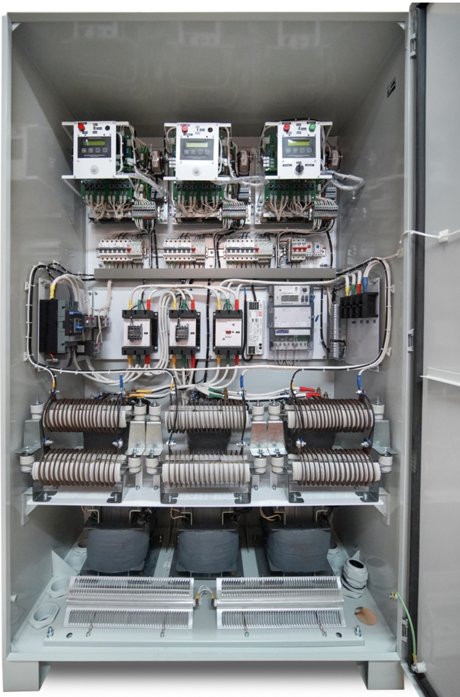
Рисунок 3.1 Внутреннее устройство
