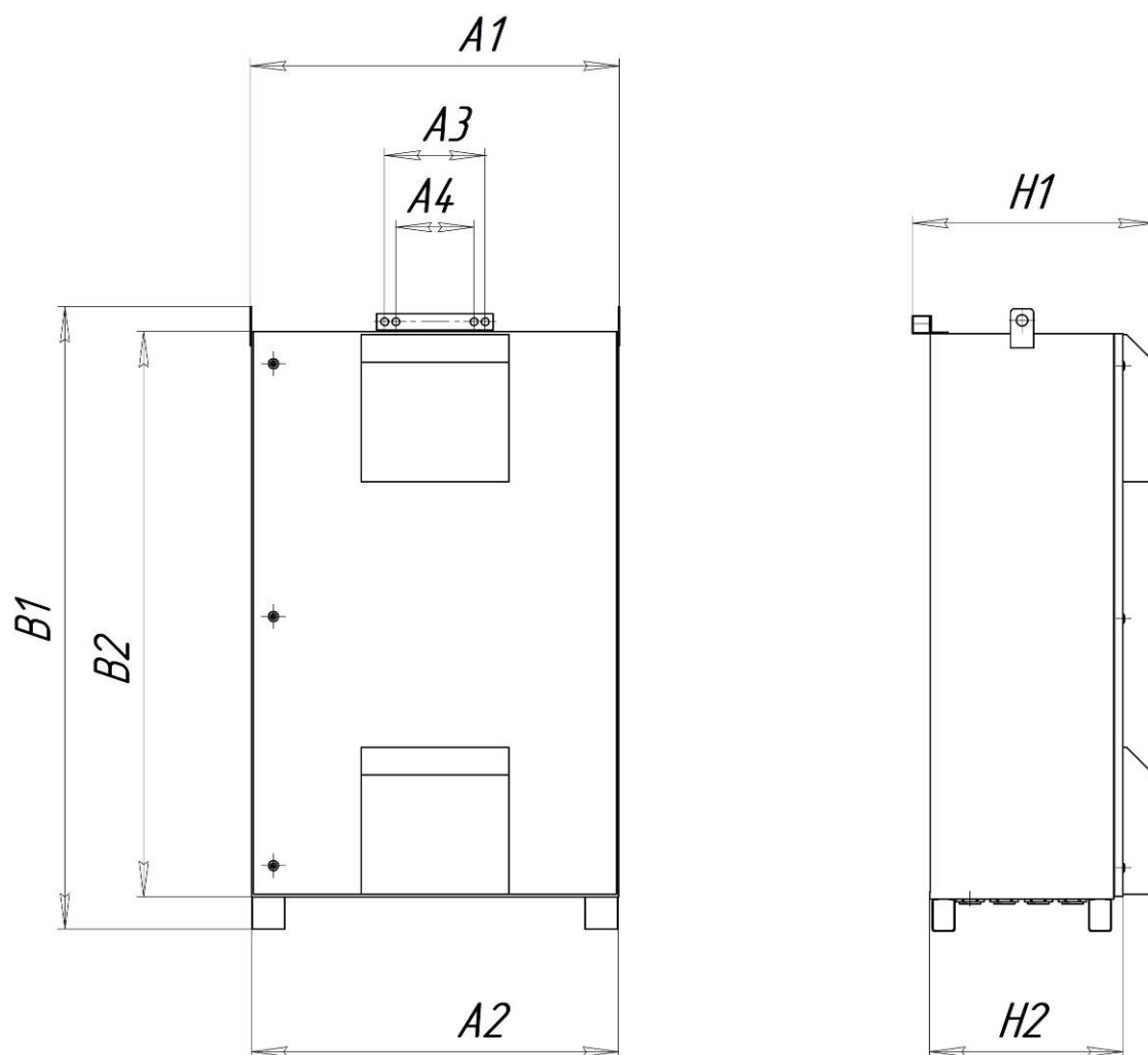
Рисунок Б1 Габаритные и присоединительные размеры СНТ-3-У
