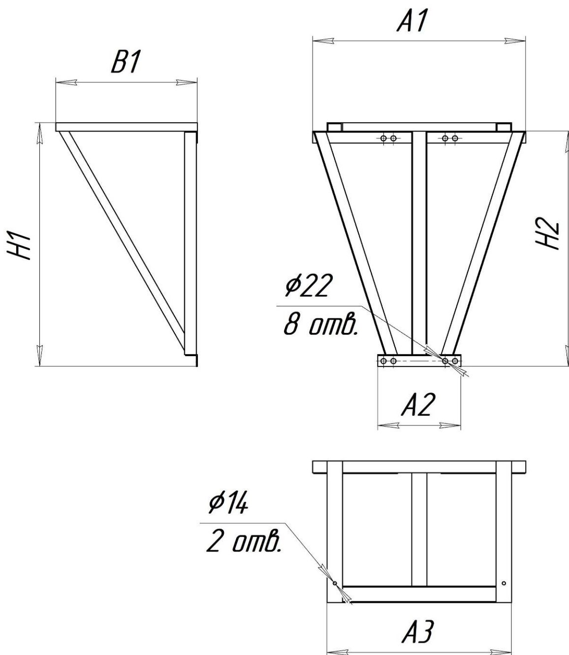
Рисунок Б2 Подвес
