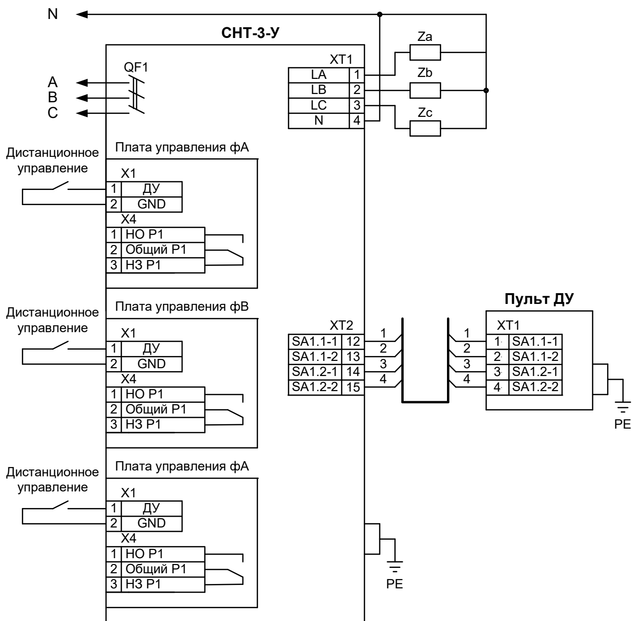
Рисунок А1 Схема внешних проводов устройства для СНТУ-1
