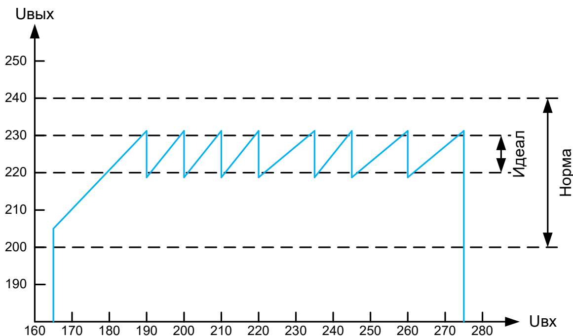
Рисунок 3.3 Примерная зависимость выходного напряжения устройства от входного
