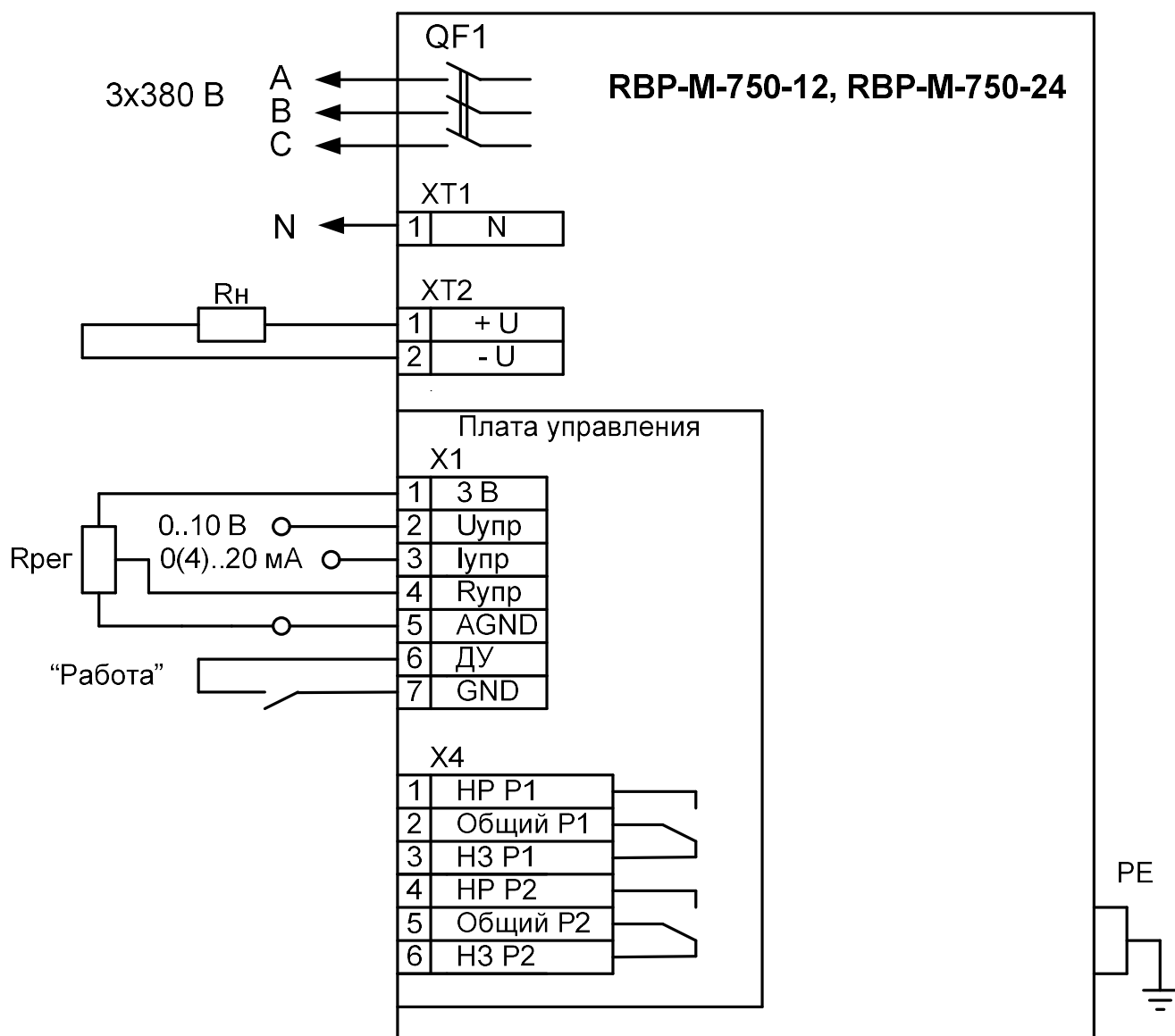
Рисунок А2 Схема подключения RBP-M-750-12, RBP-M-750-24, питание – трехфазное с нулевым проводом
