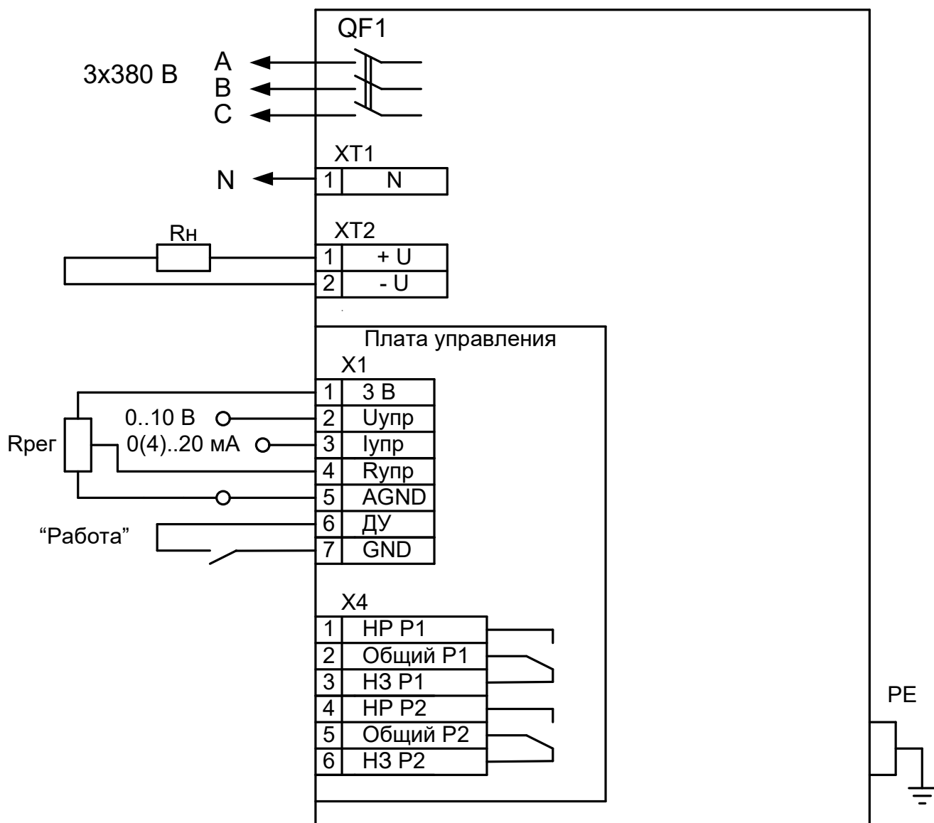
Рисунок А1 Схема подключения RBP-36-200, RBP-36-400, питание – трехфазное с нулевым проводом
