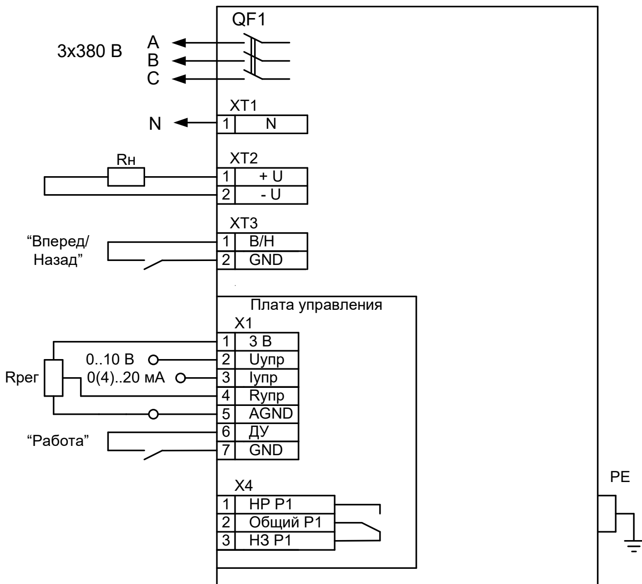
Рисунок А1 Схема подключения RBP-R-288-62, питание – трехфазное с нулевым проводом
