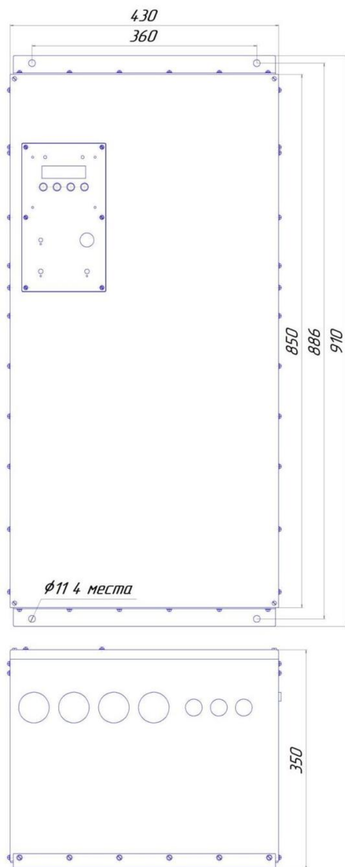
Рисунок Б3 Навесной вариант использования RBP-R-288-62. Крепежные уголки – сверху и снизу.
