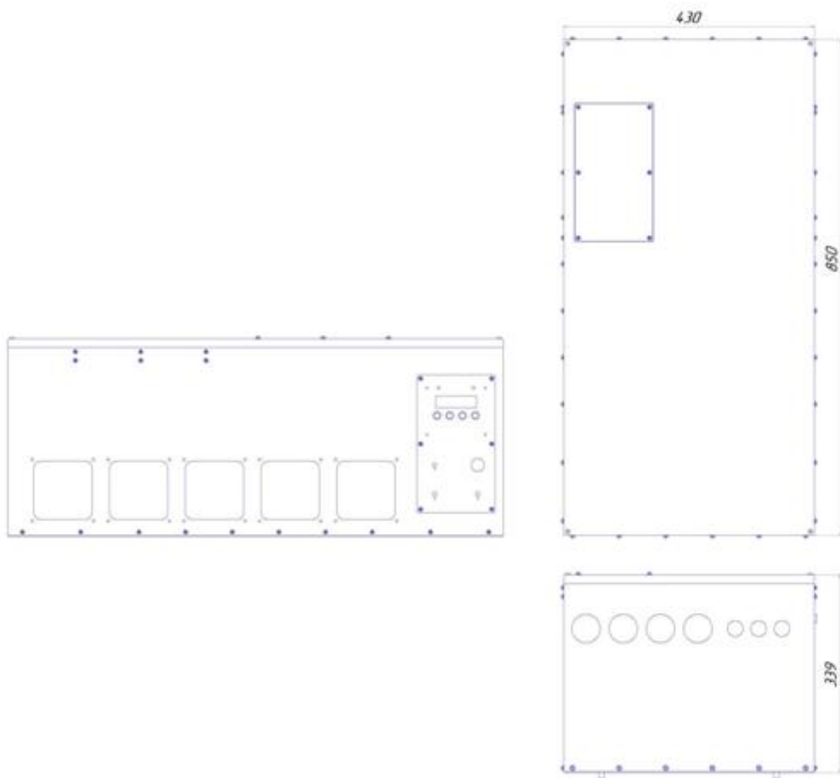
Рисунок Б4 Настольный вариант использования RBP-M-500-24, RBP-M-500-36
