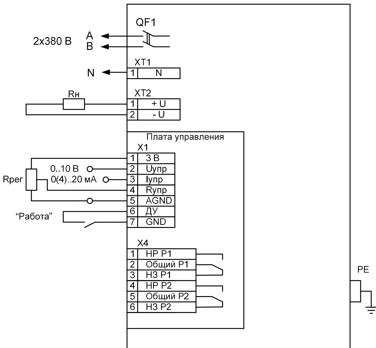
Рисунок А1 Схема подключения RBP-M-500-12, питание – двухфазное с нулевым проводом
