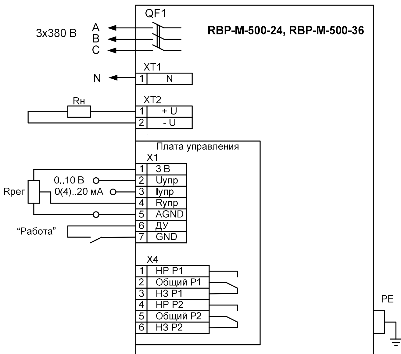
Рисунок А2 Схема подключения RBP-M-500-24, RBP-M-500-36, питание – трехфазное с нулевым проводом
