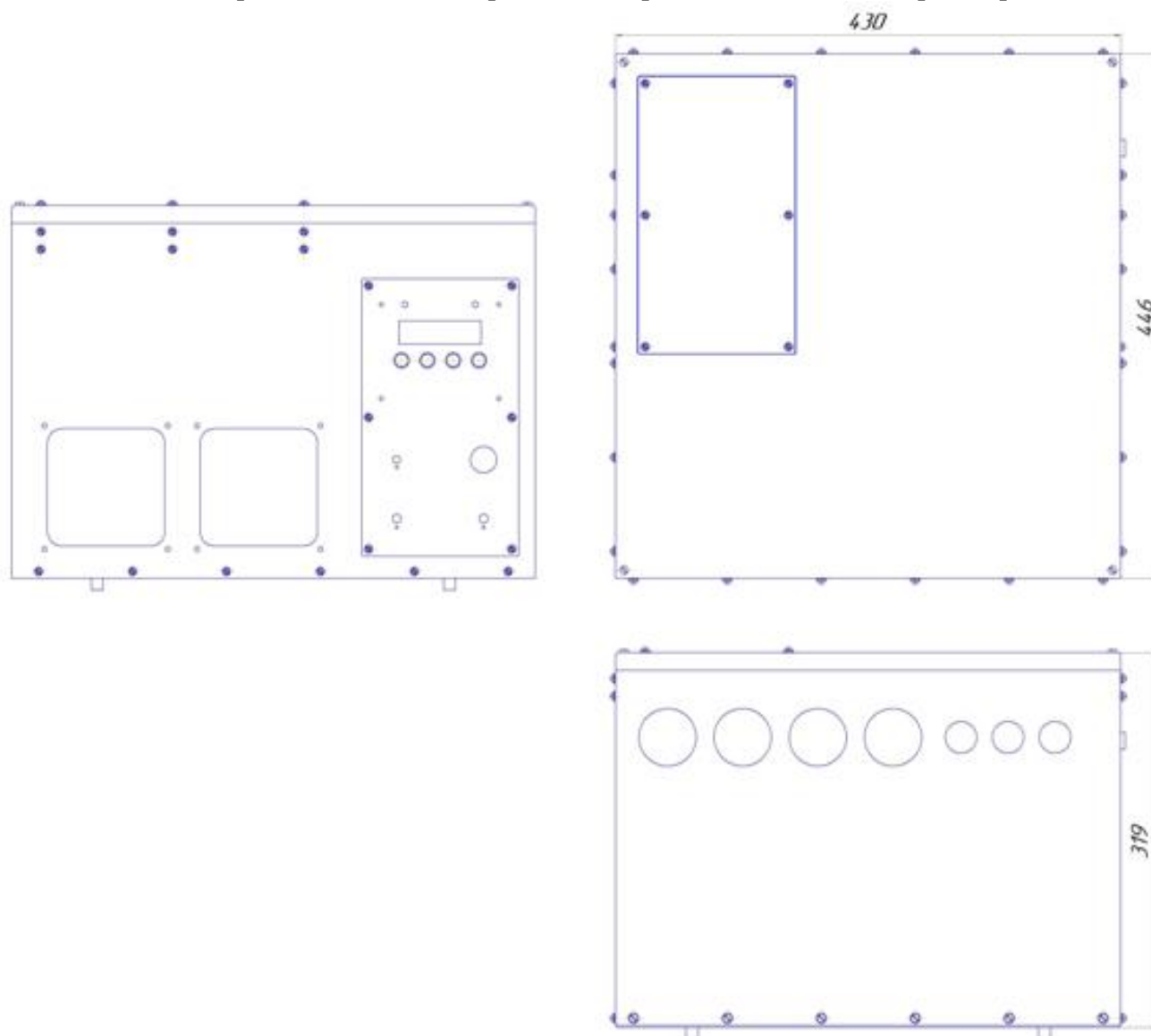
Рисунок Б1 Настольный вариант использования RBP-M-500-12
