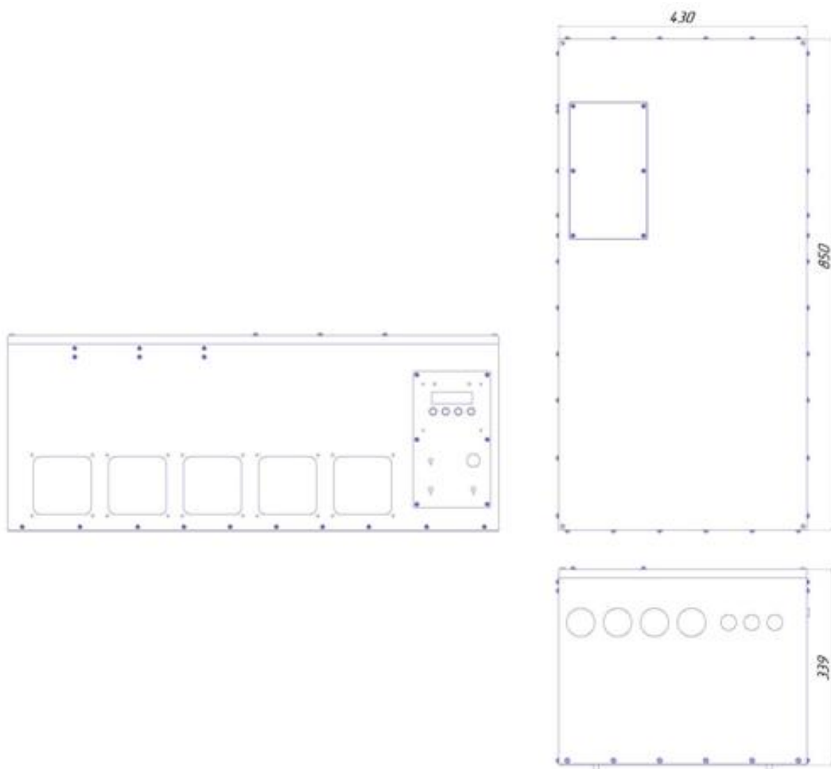
Рисунок Б4 Настольный вариант использования RBP-72-250
