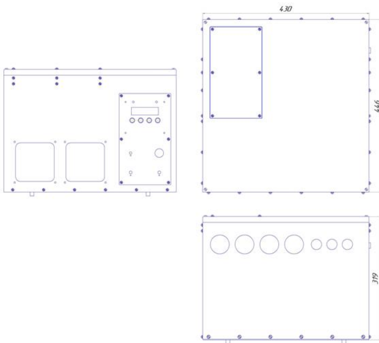
Рисунок Б1 Настольный вариант использования RBP-72-125
