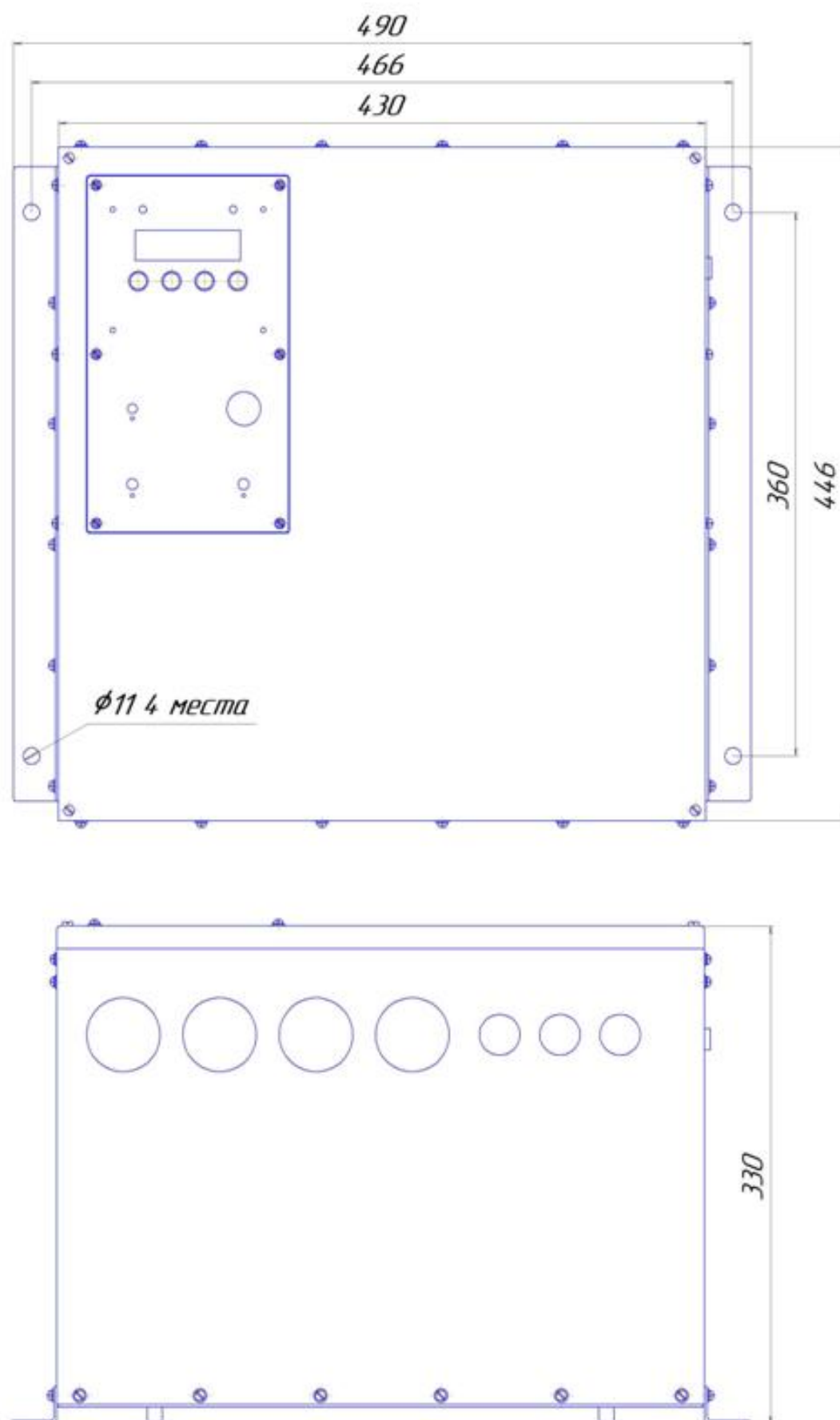
Рисунок Б2 Навесной вариант использования RBP-72-125. Крепежные уголки – слева и справа.
