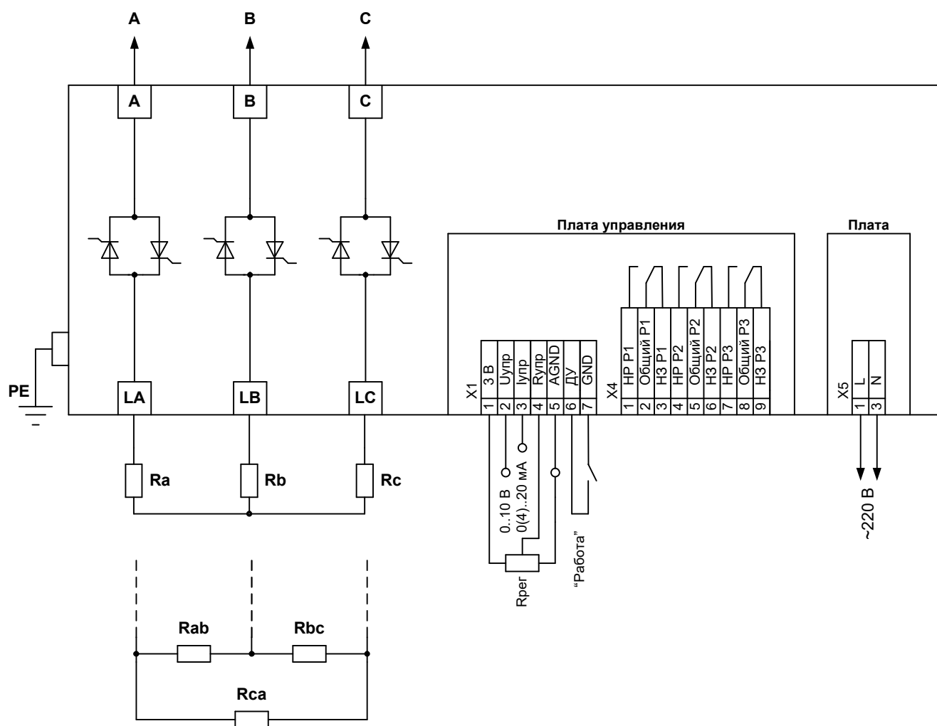
Рисунок А1 Схема подключения
