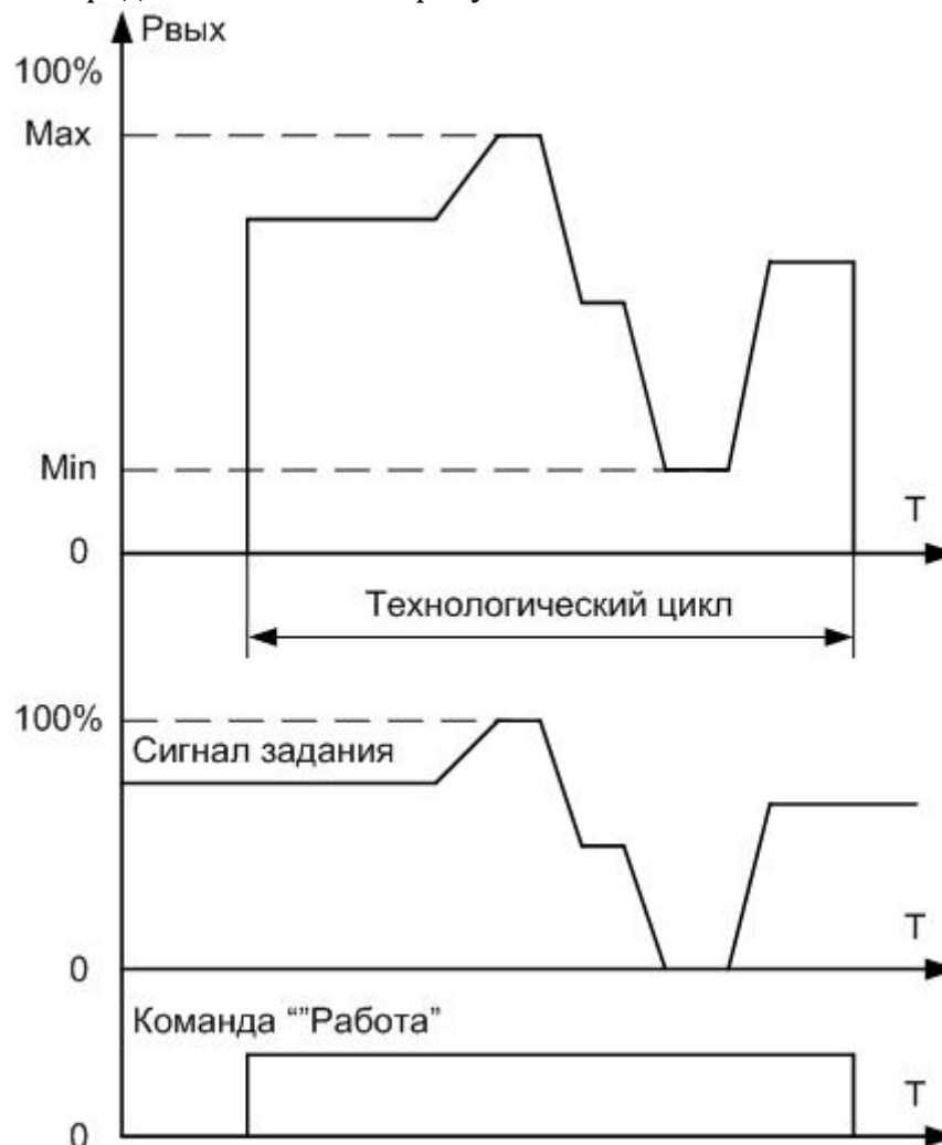
Рисунок 3.7 Рабочий цикл при регулировании методом пропуска периодов
