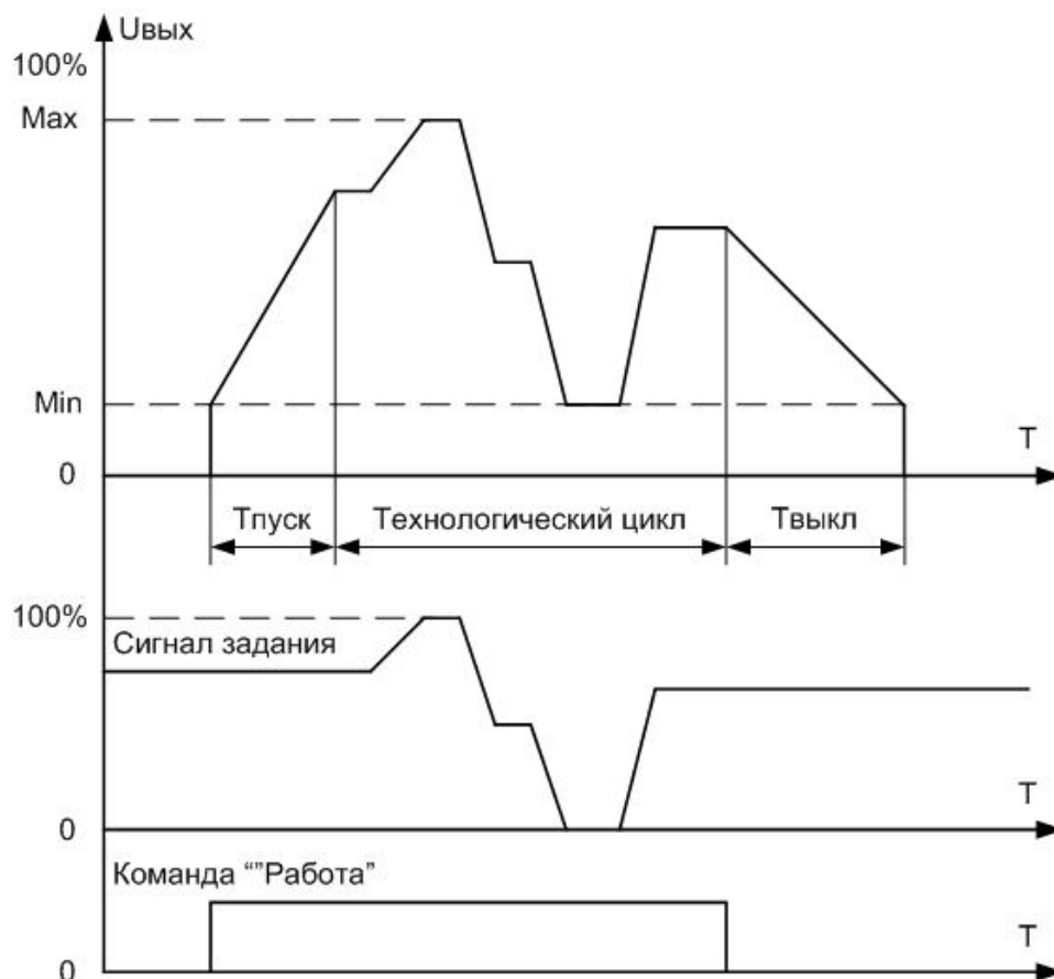
Рисунок 3.5 Рабочий цикл при фазовом методе регулирования
