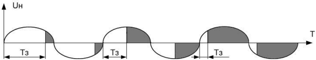
Рисунок 3.4 Выходное напряжение при фазовом способе регулирования
