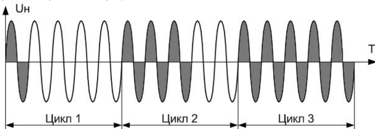
Рисунок 3.6 Выходное напряжение при регулировании методом пропуска периодов
