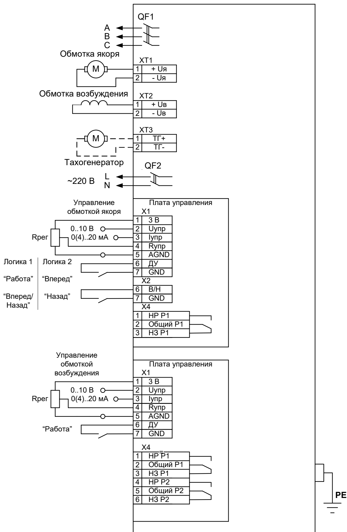
Рисунок А1 Схема подключения
