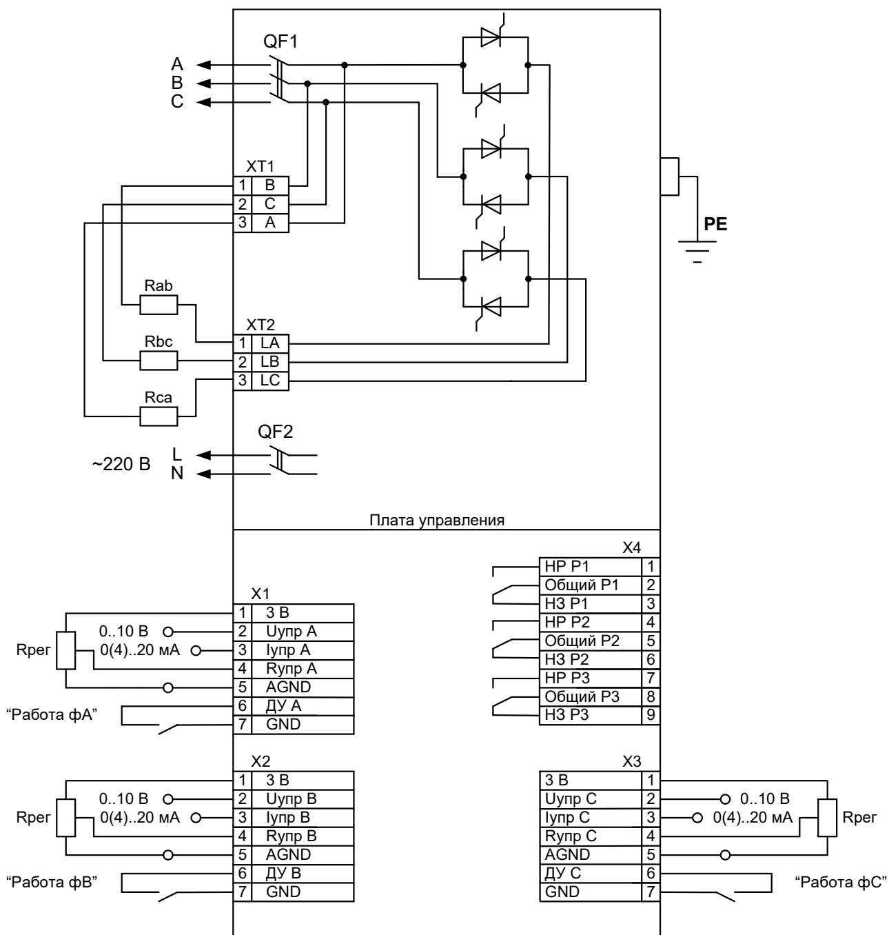
Рисунок А1 Схема подключения нагрузки – “разомкнутый треугольник”
