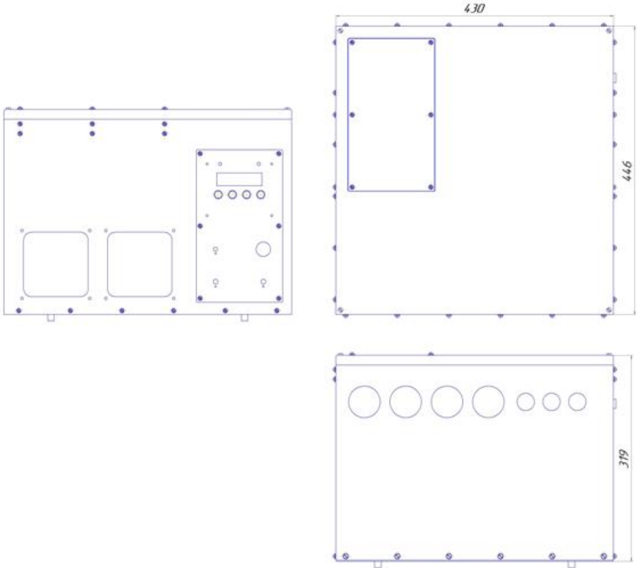
Рисунок Б1 Настольный вариант использования RBP-R-M-750-12
