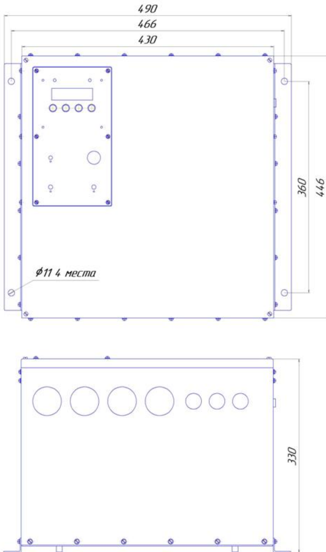
Рисунок Б2 Навесной вариант использования RBP-R-M-750-12. Крепежные уголки – слева и справа.
