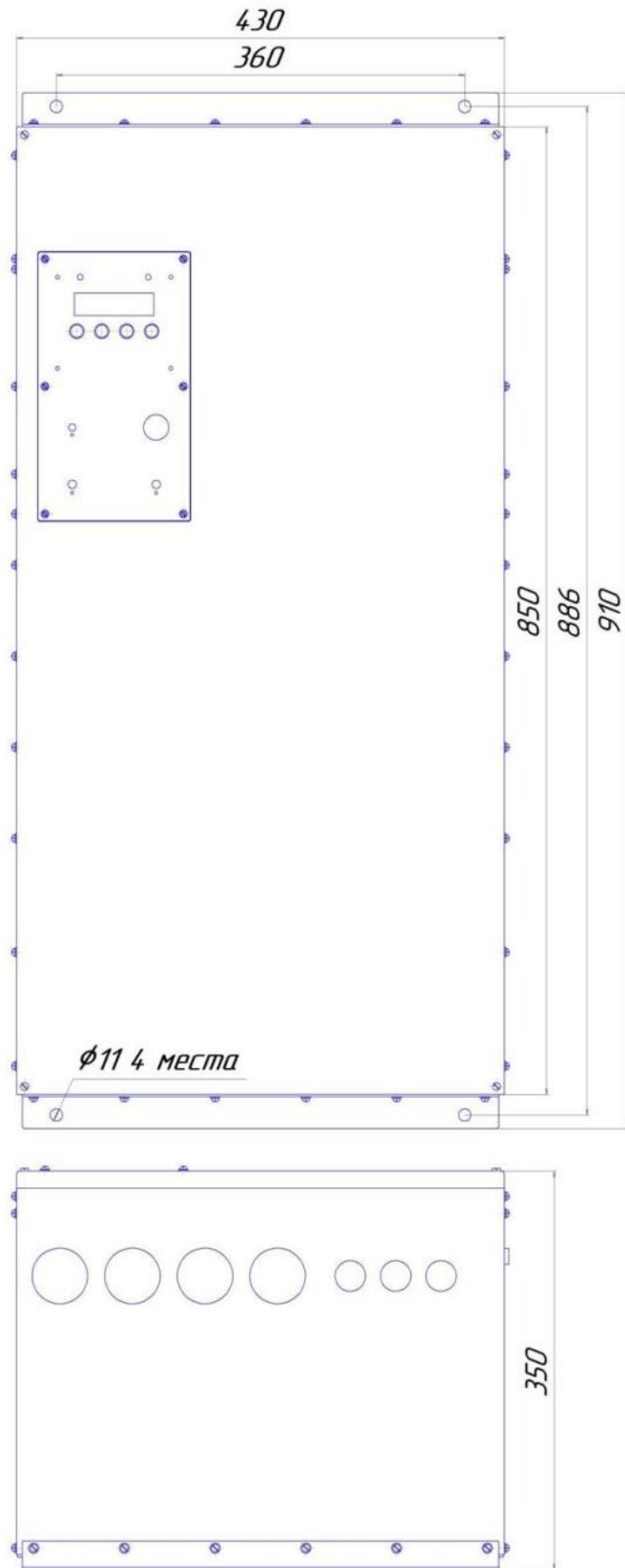
Рисунок Б6 Навесной вариант использования RBP-R-M-750-24. Крепежные уголки – сверху и снизу.
