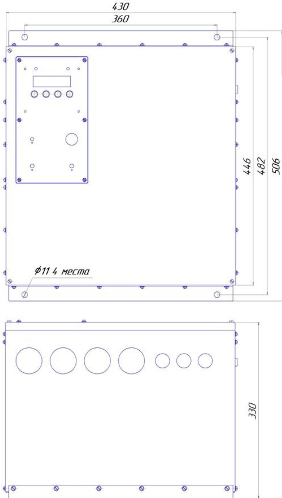
Рисунок Б3 Навесной вариант использования RBP-R-M-750-12. Крепежные уголки – сверху и снизу.
