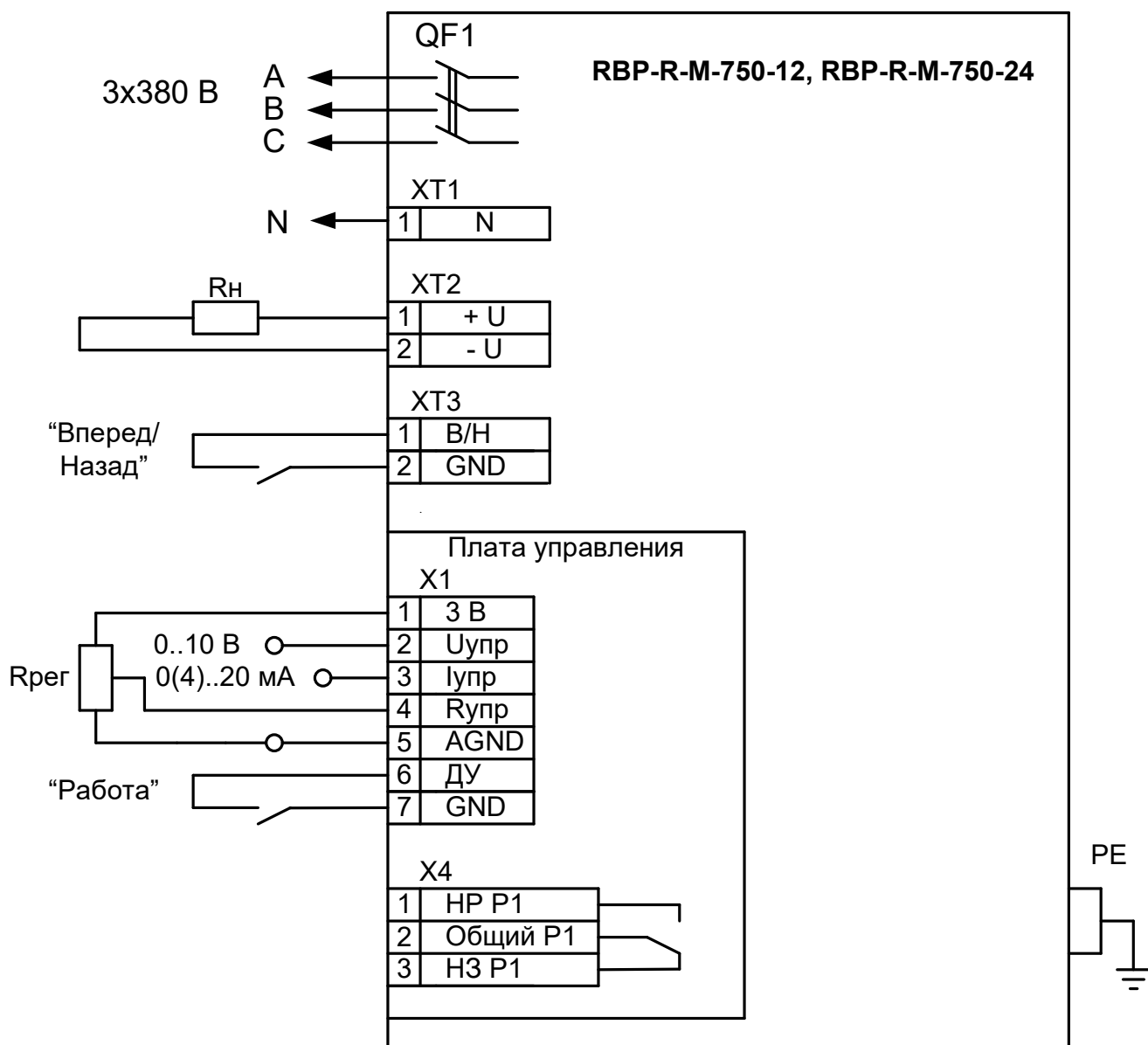
Рисунок А2 Схема подключения RBP-R-M-750-12, RBP-R-M-750-24, питание – трехфазное с нулевым проводом
