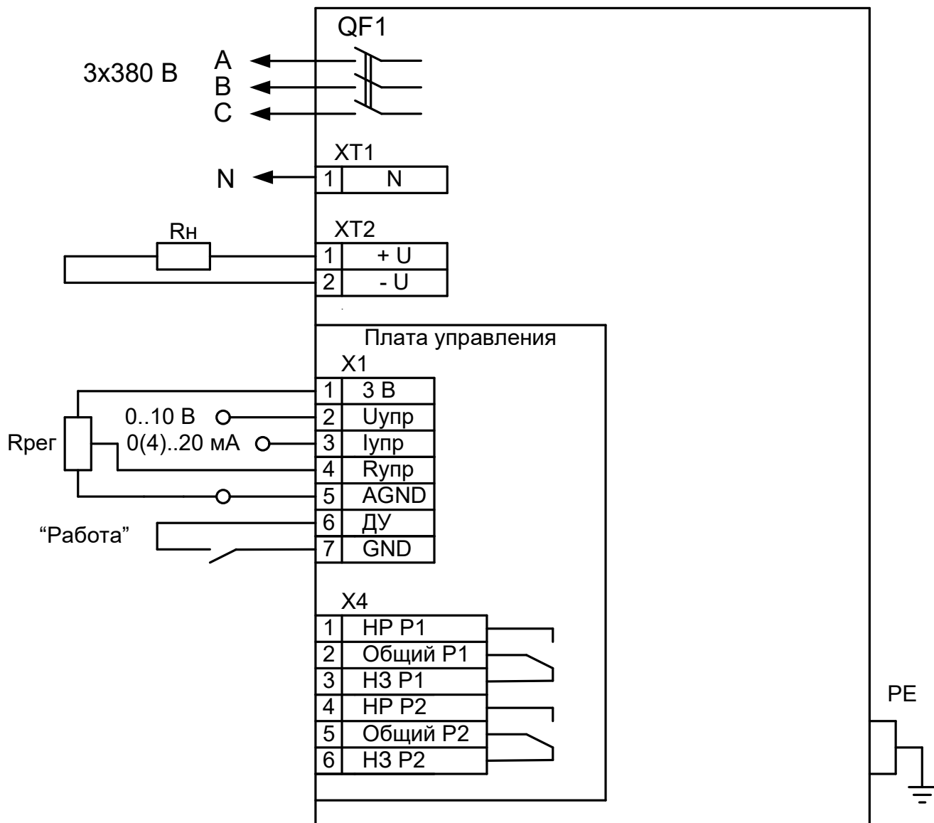
Рисунок А1 Схема подключения RBP-120-125, питание – трехфазное с нулевым проводом
