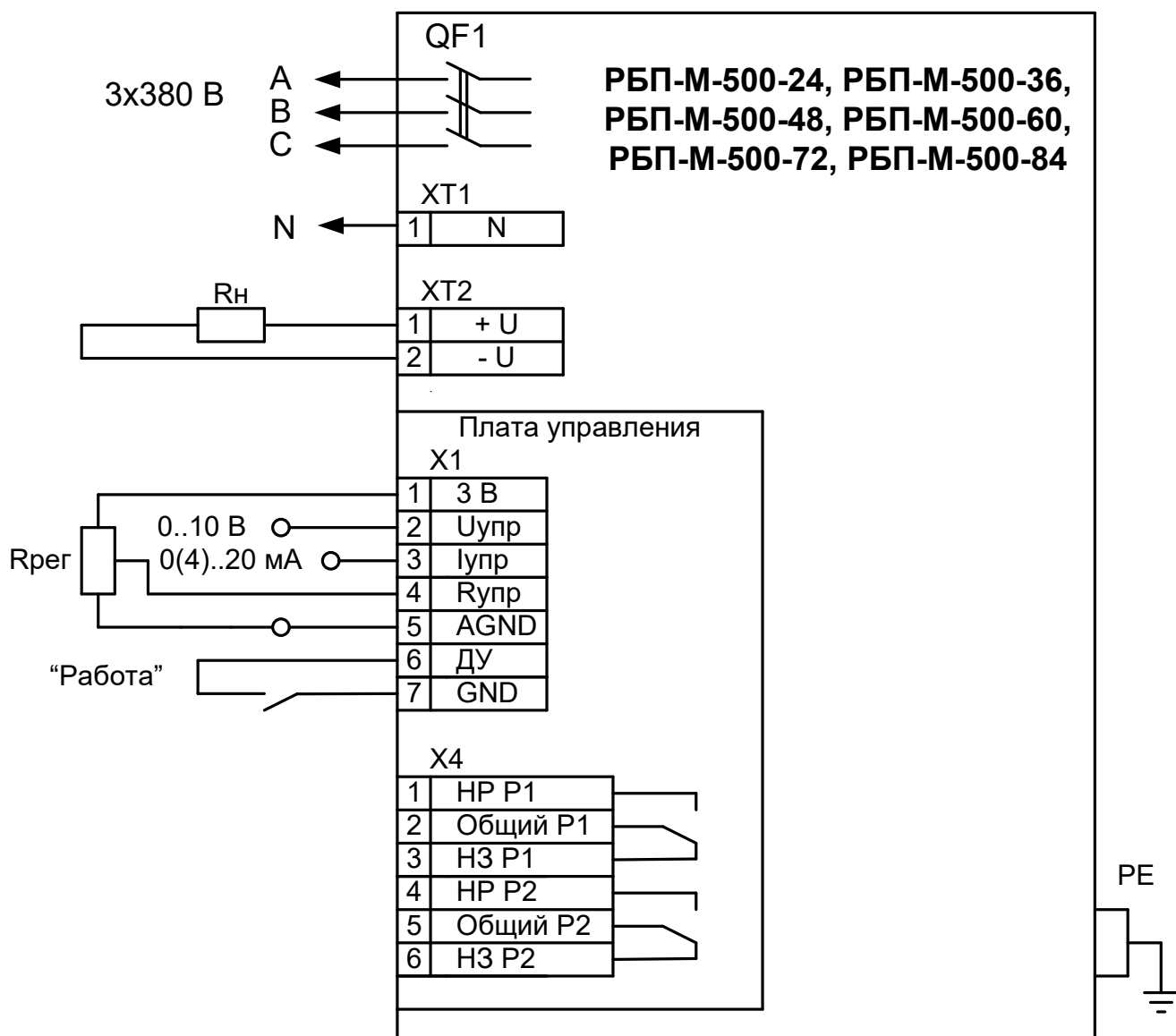
Рисунок А2 Схема подключения РБП-М-500-24, РБП-М-500-36, РБП-М-500-48, РБП-М-500-60, РБП-М-500-72, РБП-М-500-84, питание – трехфазное с нулевым проводом
