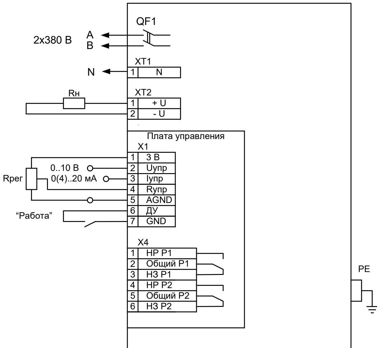
Рисунок А1 Схема подключения РБП-М-500-12, питание – двухфазное с нулевым проводом
