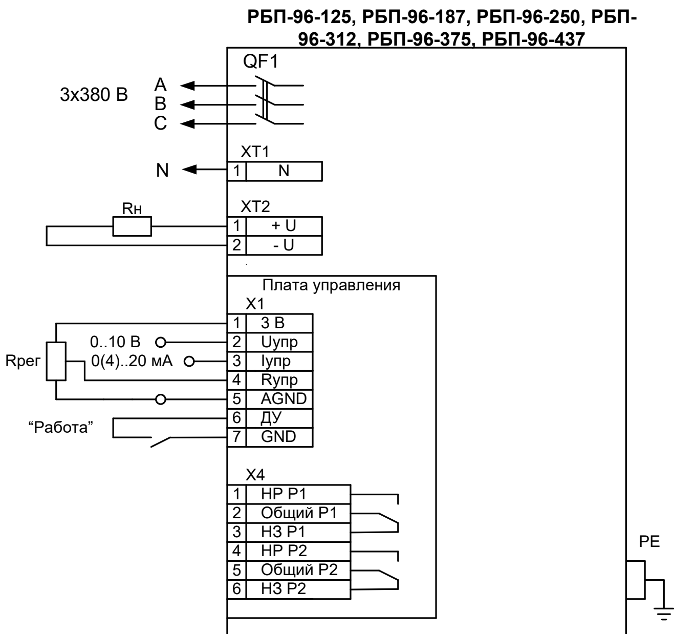
Рисунок А3 Схема подключения РБП-96-125, РБП-96-187, РБП-96-250, РБП-96-312, РБП-96-375, РБП-96-437, питание – трехфазное с нулевым проводом
