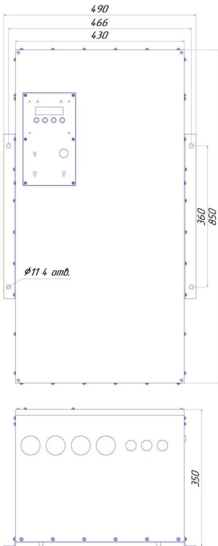
Рисунок Б8 Навесной вариант использования RBP-M-120-100, RBP-M-120-125, RBP-M-120-150. Крепежные уголки – слева и справа.
