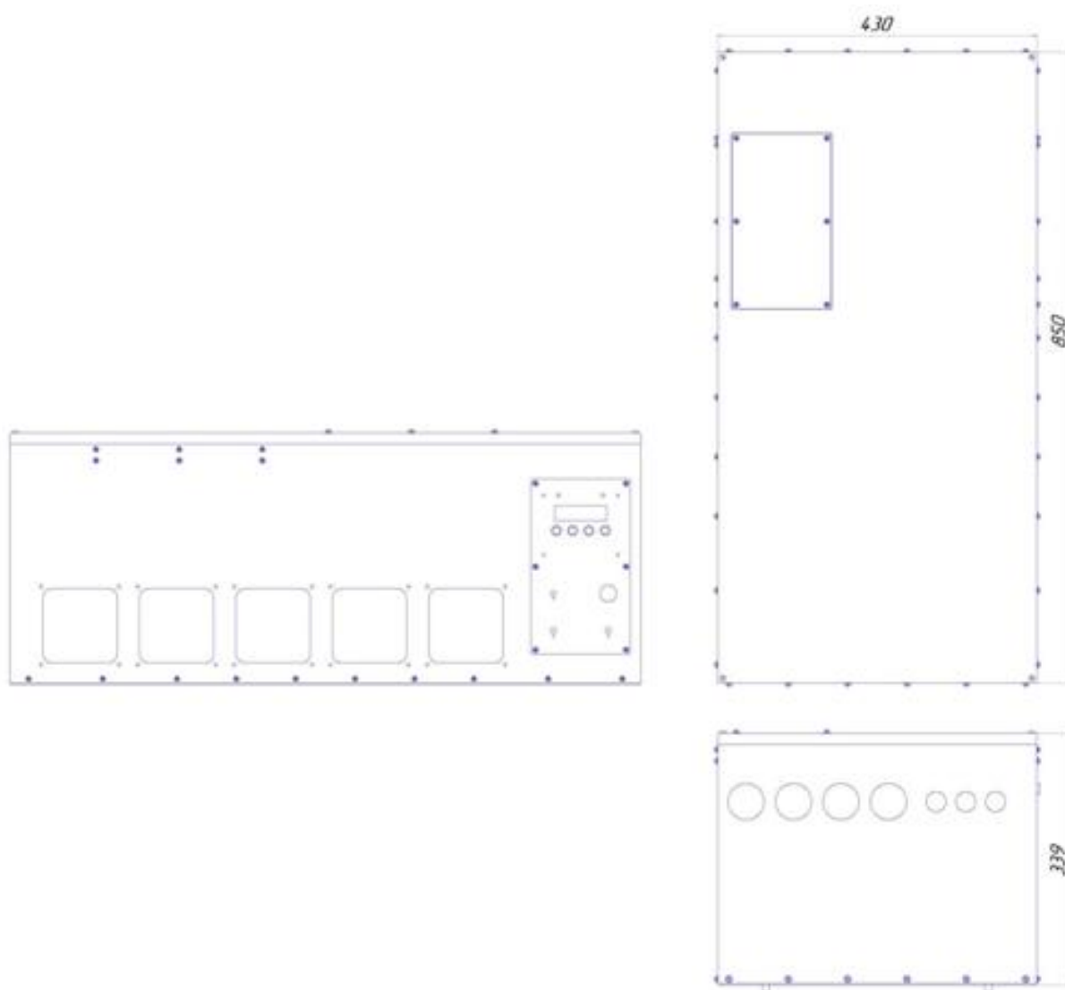
Рисунок Б7 Настольный вариант использования RBP-M-120-100, RBP-M-120-125, RBP-M-120-150
