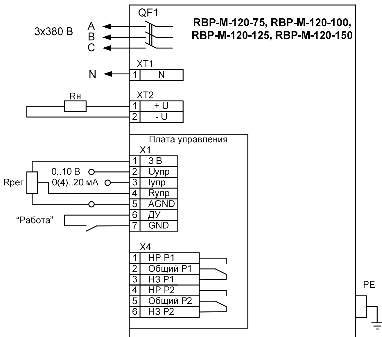
Рисунок А3 Схема подключения RBP-M-120-75, RBP-M-120-100, RBP-M-120-125, RBP-M-120-150, питание – трехфазное с нулевым проводом
