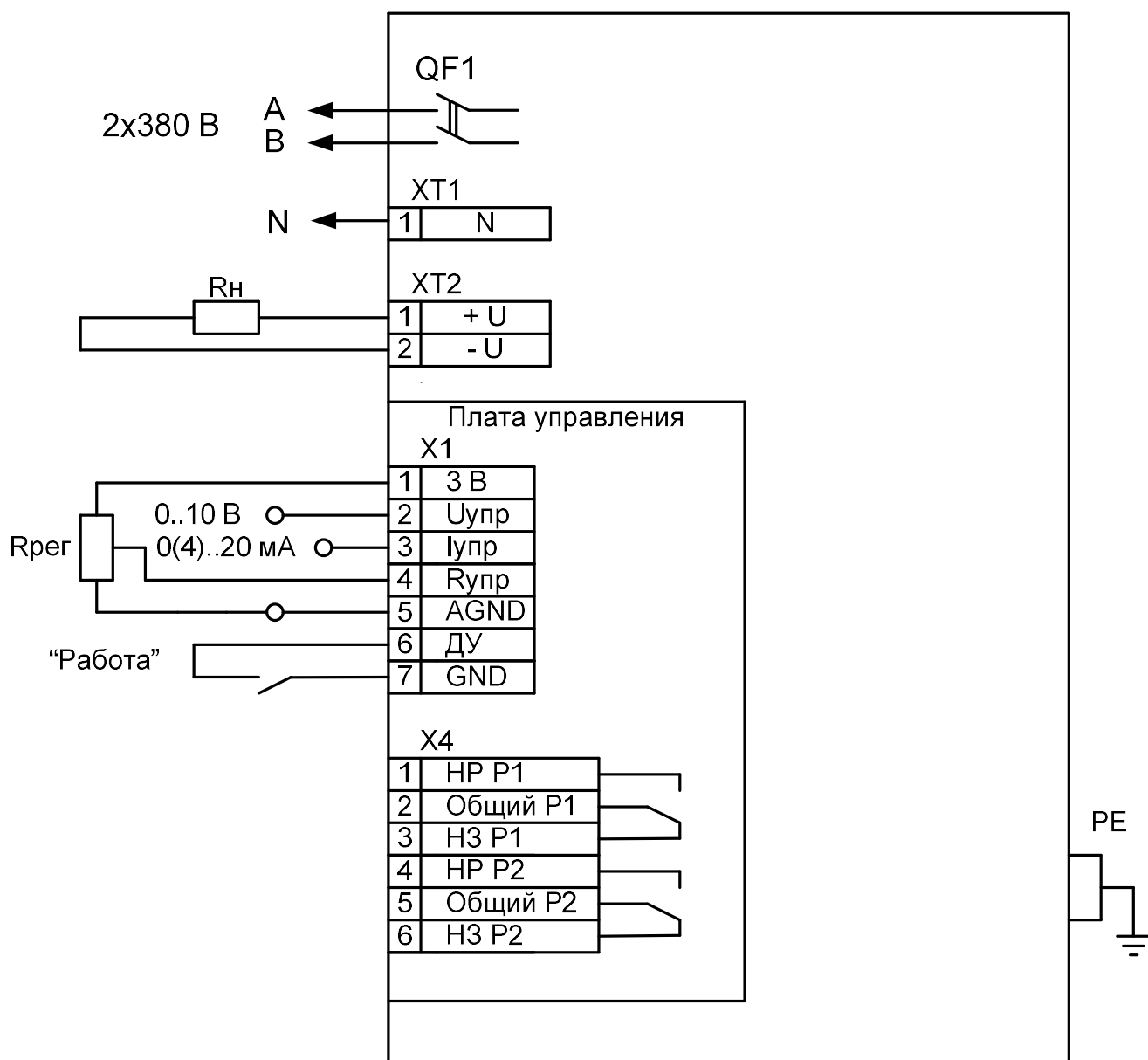
Рисунок А2 Схема подключения RBP-M-120-50, питание – двухфазное с нулевым проводом
