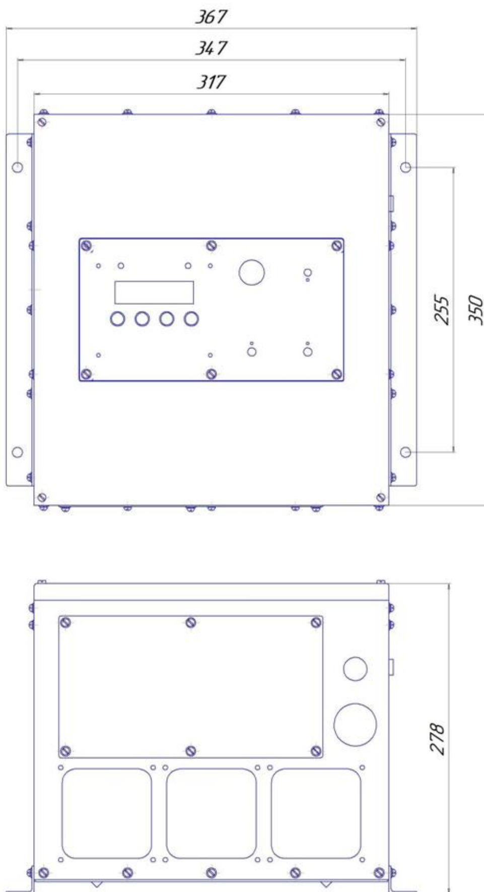
Рисунок Б2 Навесной вариант использования RBP-M-120-25. Крепежные уголки – слева и справа.
