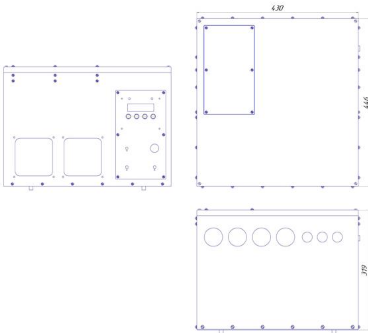
Рисунок Б4 Настольный вариант использования RBP-M-120-50, RBP-M-120-75
