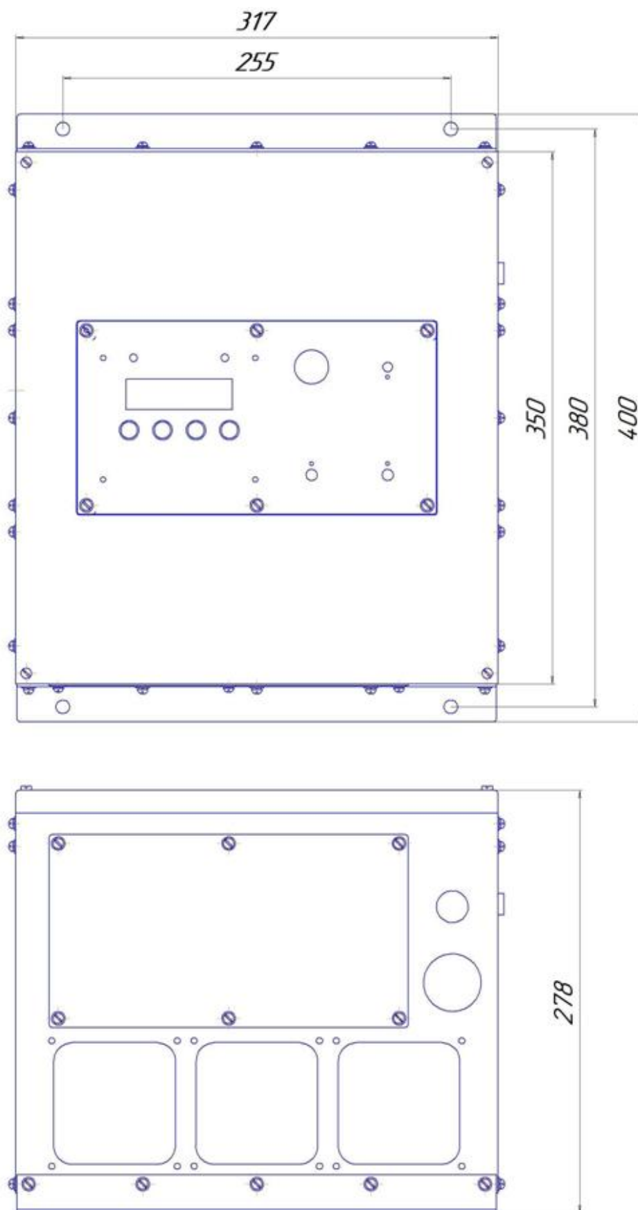
Рисунок Б3 Навесной вариант использования RBP-M-120-25. Крепежные уголки – сверху и снизу.
