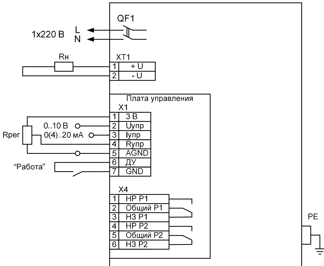
Рисунок А1 Схема подключения RBP-M-120-25, питание - однофазное
