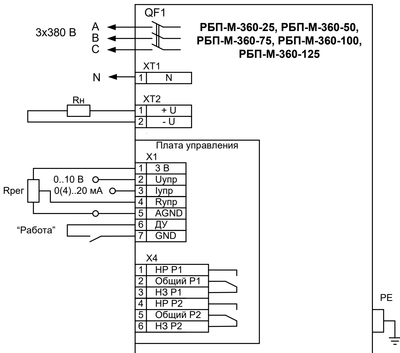
Рисунок А1 Схема подключения РБП-М-360-25, РБП-М-360-50, РБП-М-360-75, РБП-М-360-100, РБП-М-360-125, питание – трехфазное с нулевым проводом
