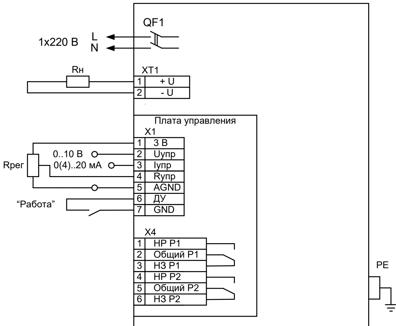
Рисунок А1 Схема подключения РБП-М-120-25, питание - однофазное
