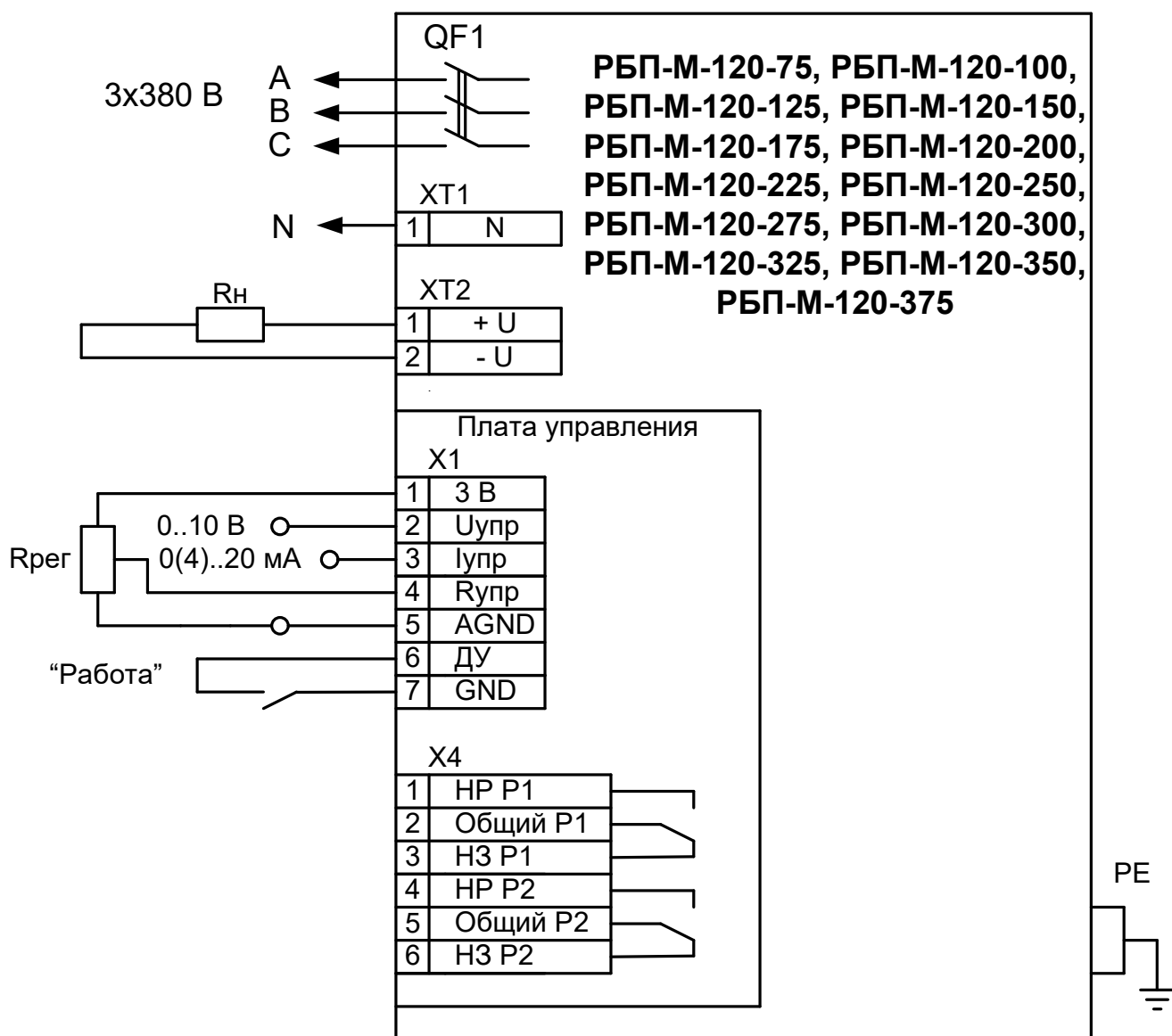
Рисунок А3 Схема подключения РБП-М-120-75, РБП-М-120-100, РБП-М-120-125, РБП-М-120-150, РБП-М-120-175, РБП-М-120-200, РБП-М-120-225, РБП-М-120-250, РБП-М-120-275, РБП-М-120-300, РБП-М-120-325, РБП-М-120-350, РБП-М-120-375, питание – трехфазное с нулевым проводом
