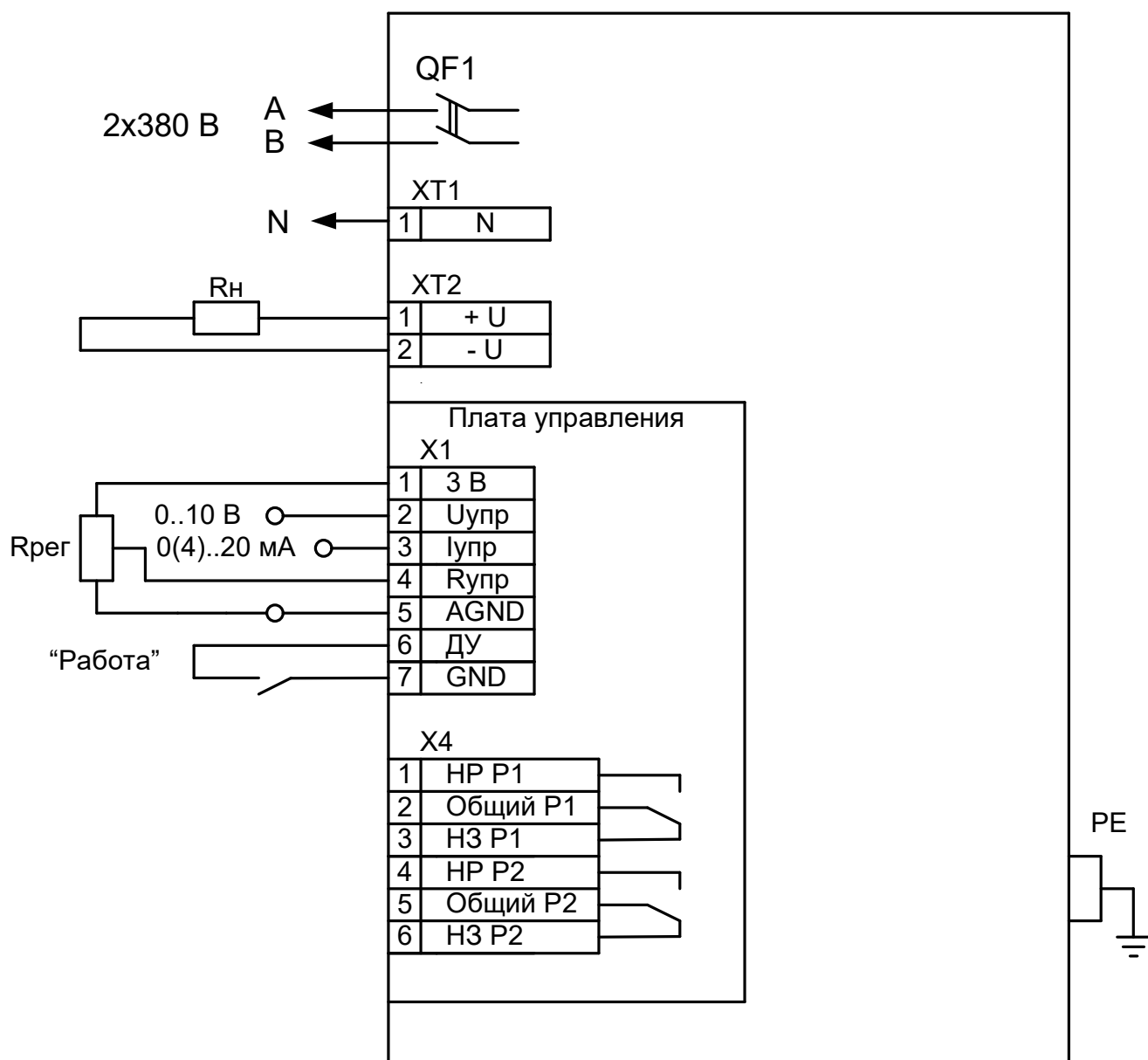
Рисунок А2 Схема подключения РБП-М-120-50, питание – двухфазное с нулевым проводом
