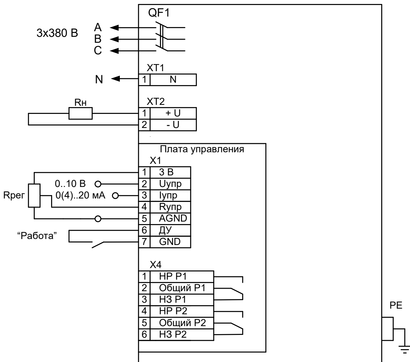
Рисунок А3 Схема подключения РБП-336-62, РБП-336-125, питание – трехфазное с нулевым проводом
