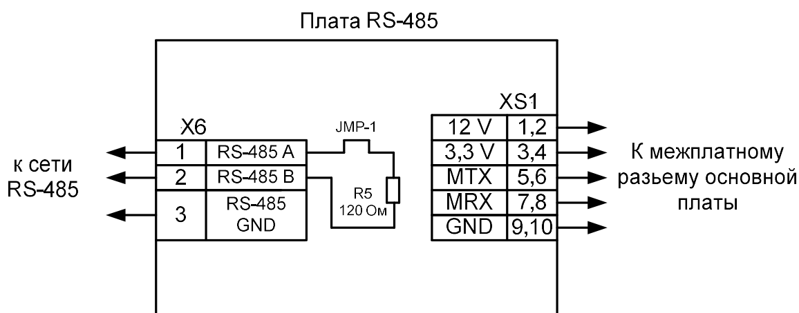
Рисунок 3.2 Схема подключения платы
