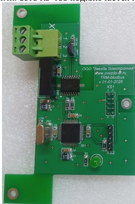
Рисунок 3.1 Внешний вид платы RS-485
