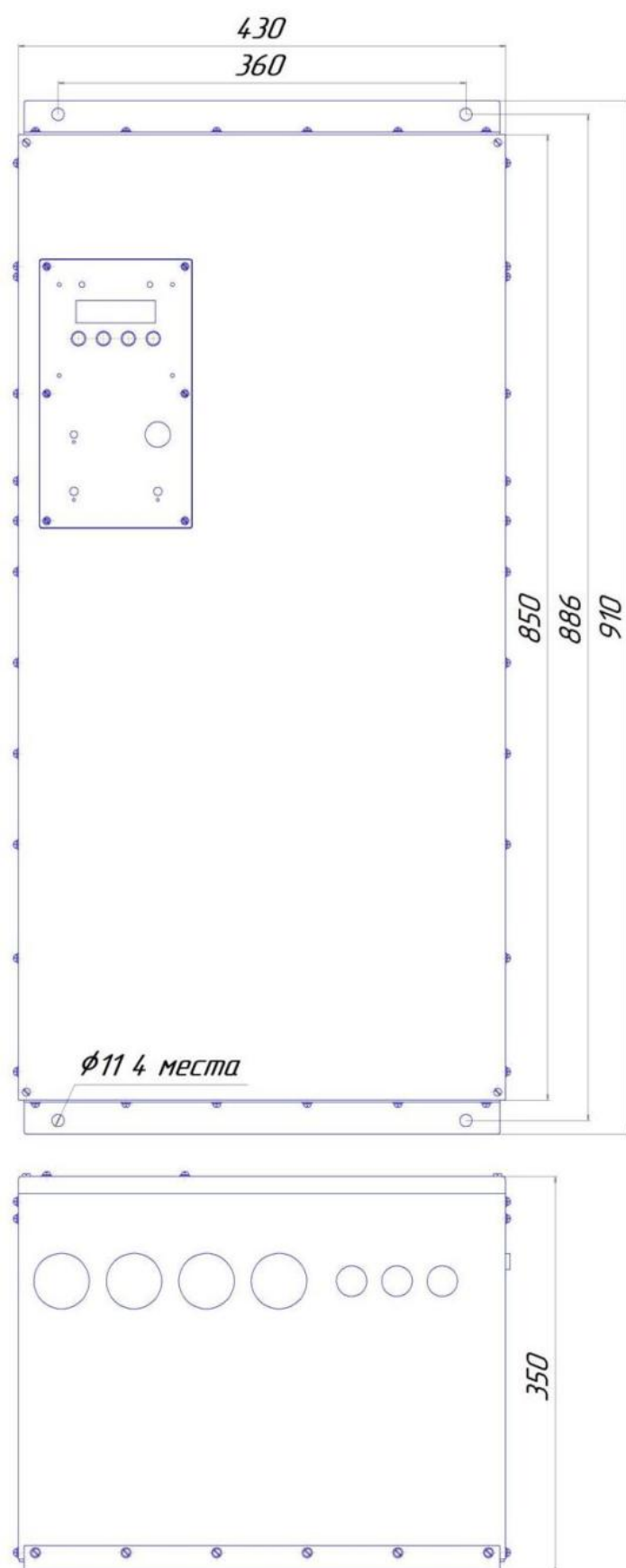
Рисунок Б3 Навесной вариант использования RBP-192-62. Крепежные уголки – сверху и снизу.
