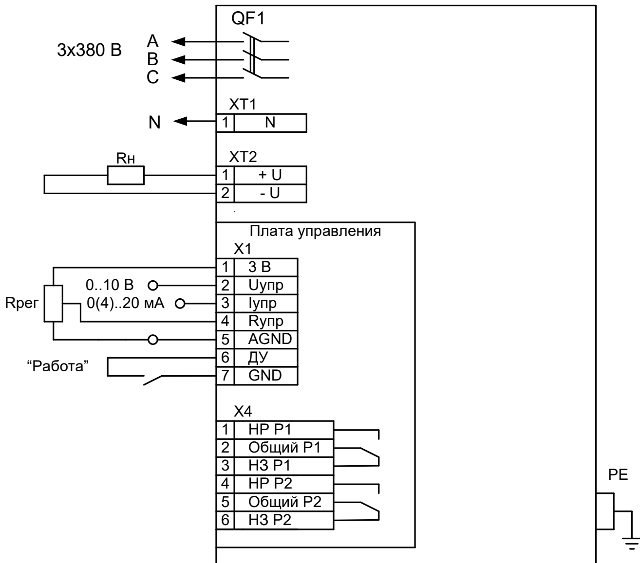
Рисунок А1 Схема подключения RBP-192-62, питание – трехфазное с нулевым проводом
