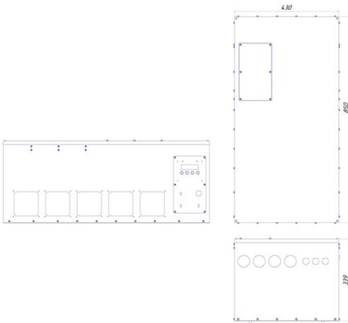
Рисунок Б1 Настольный вариант использования RBP-192-62
