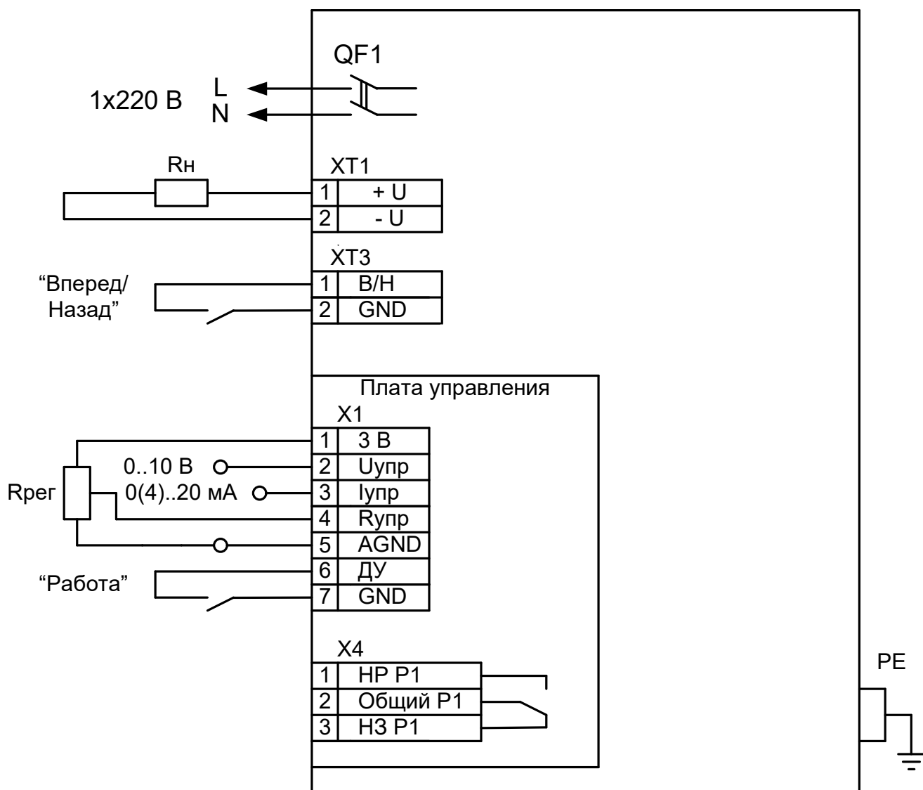
Рисунок А1 Схема подключения RBP-R-48-62
