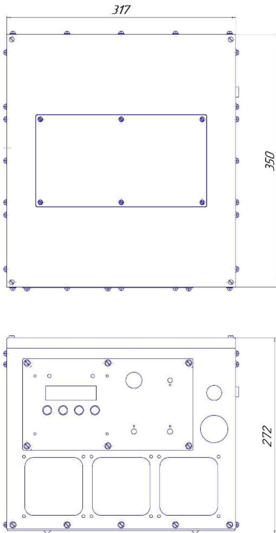
Рисунок Б1 Настольный вариант использования RBP-R-48-62
