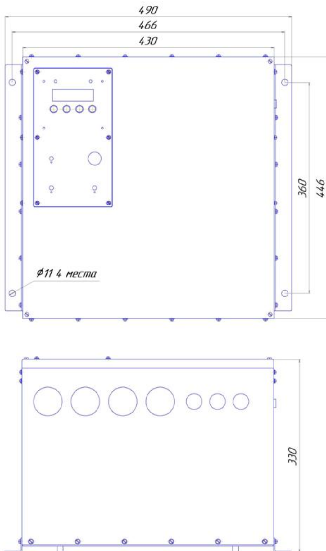
Рисунок Б5 Навесной вариант использования RBP-R-48-125. Крепежные уголки – слева и справа.
