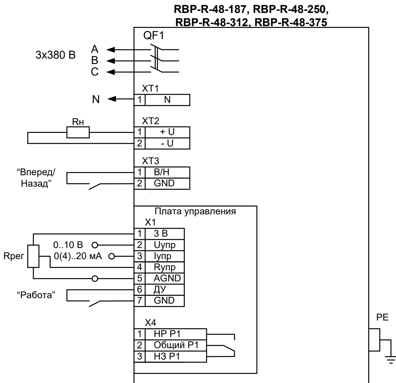
Рисунок А3 Схема подключения RBP-R-48-187, RBP-R-48-250, RBP-R-48-312, RBP-R-48-375, питание – трехфазное с нулевым проводом
