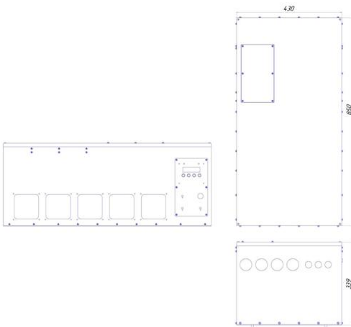
Рисунок Б1 Настольный вариант использования RBP-R-120-125
