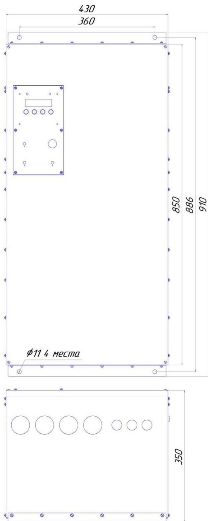
Рисунок Б3 Навесной вариант использования RBP-R-120-125. Крепежные уголки – сверху и снизу.
