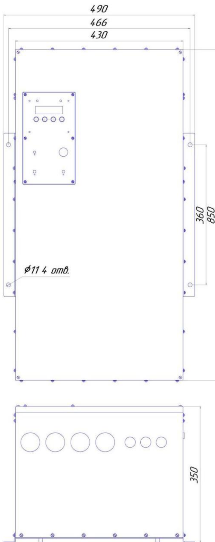
Рисунок Б2 Навесной вариант использования RBP-R-120-125. Крепежные уголки – слева и справа.
