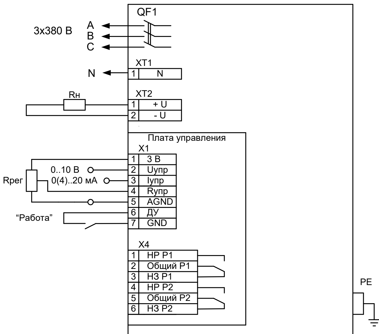
Рисунок А2 Схема подключения RBP-96-125, RBP-96-187, питание – трехфазное с нулевым проводом
