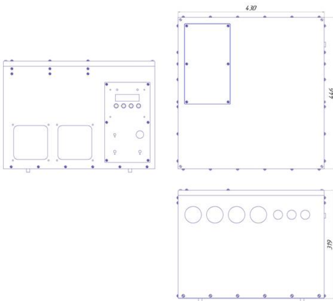
Рисунок Б1 Настольный вариант использования RBP-96-62
