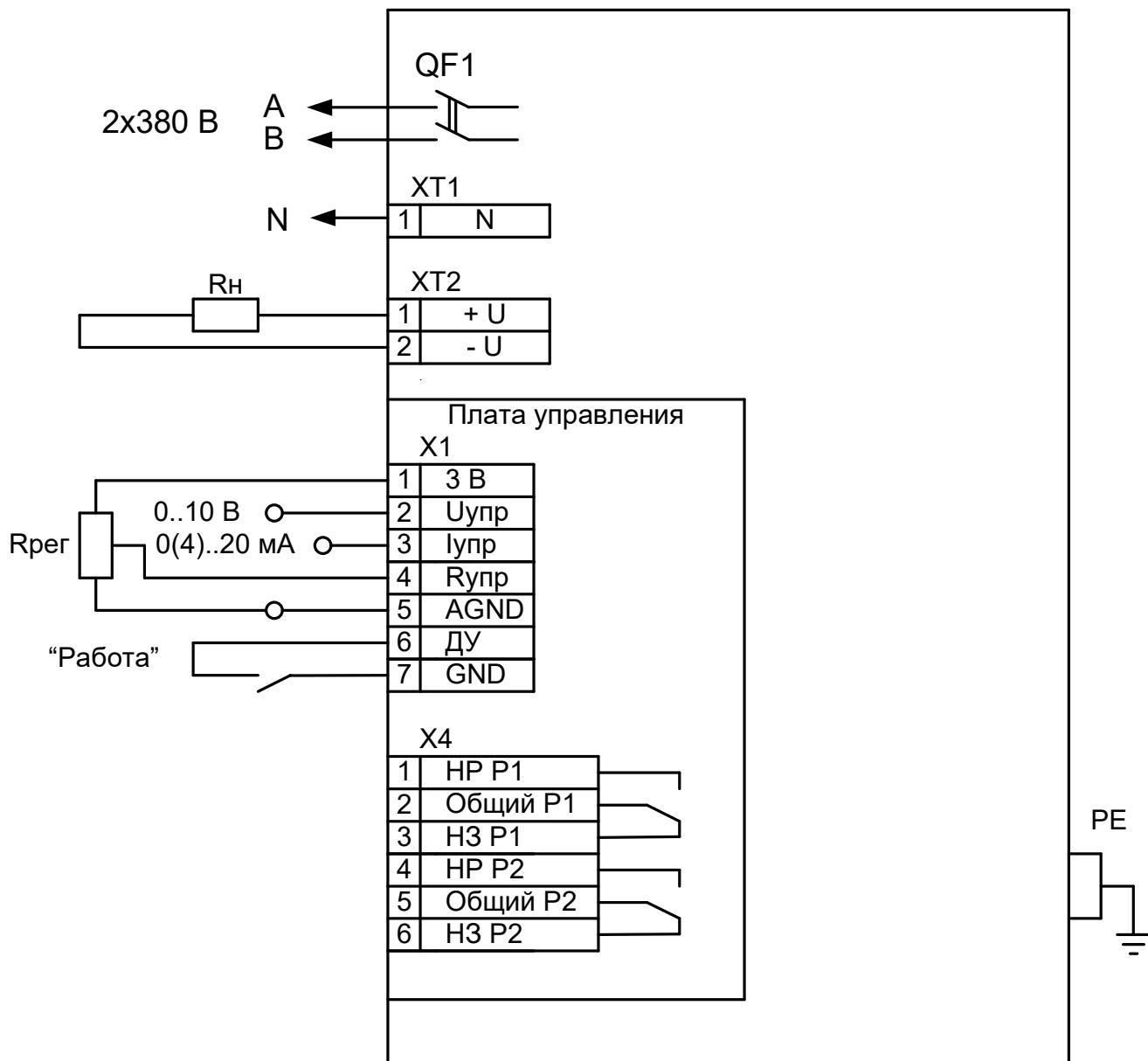
Рисунок А1 Схема подключения RBP-96-62, питание – двухфазное с нулевым проводом
