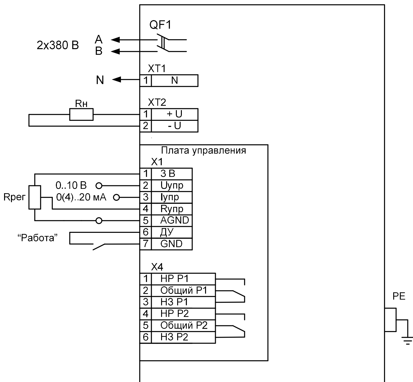
Рисунок А2 Схема подключения RBP-M-250-24, питание – двухфазное с нулевым проводом
