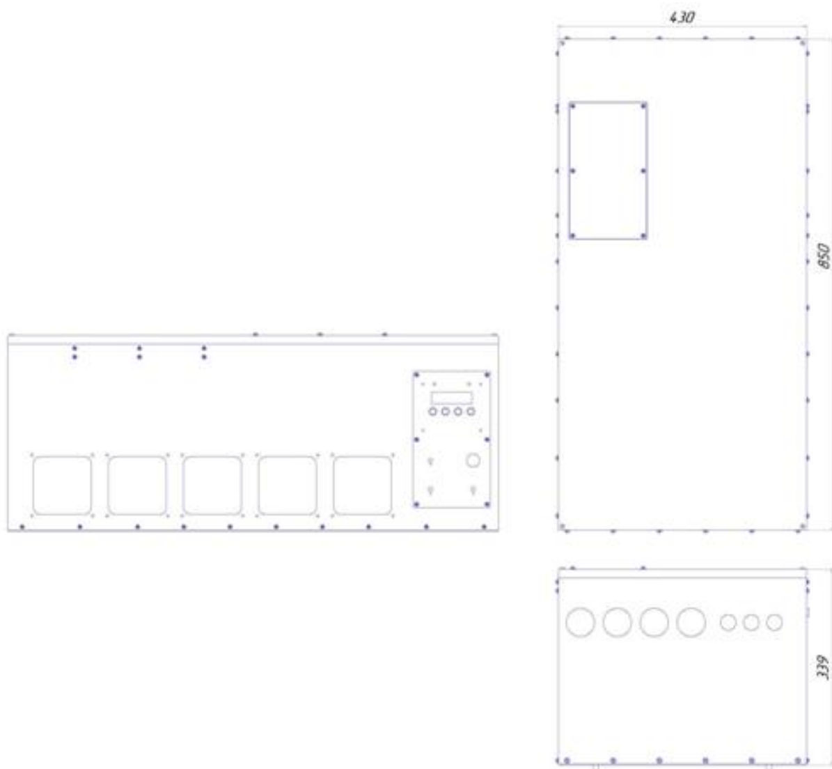
Рисунок Б7 Настольный вариант использования RBP-M-250-48, RBP-M-250-60, RBP-M-250-72
