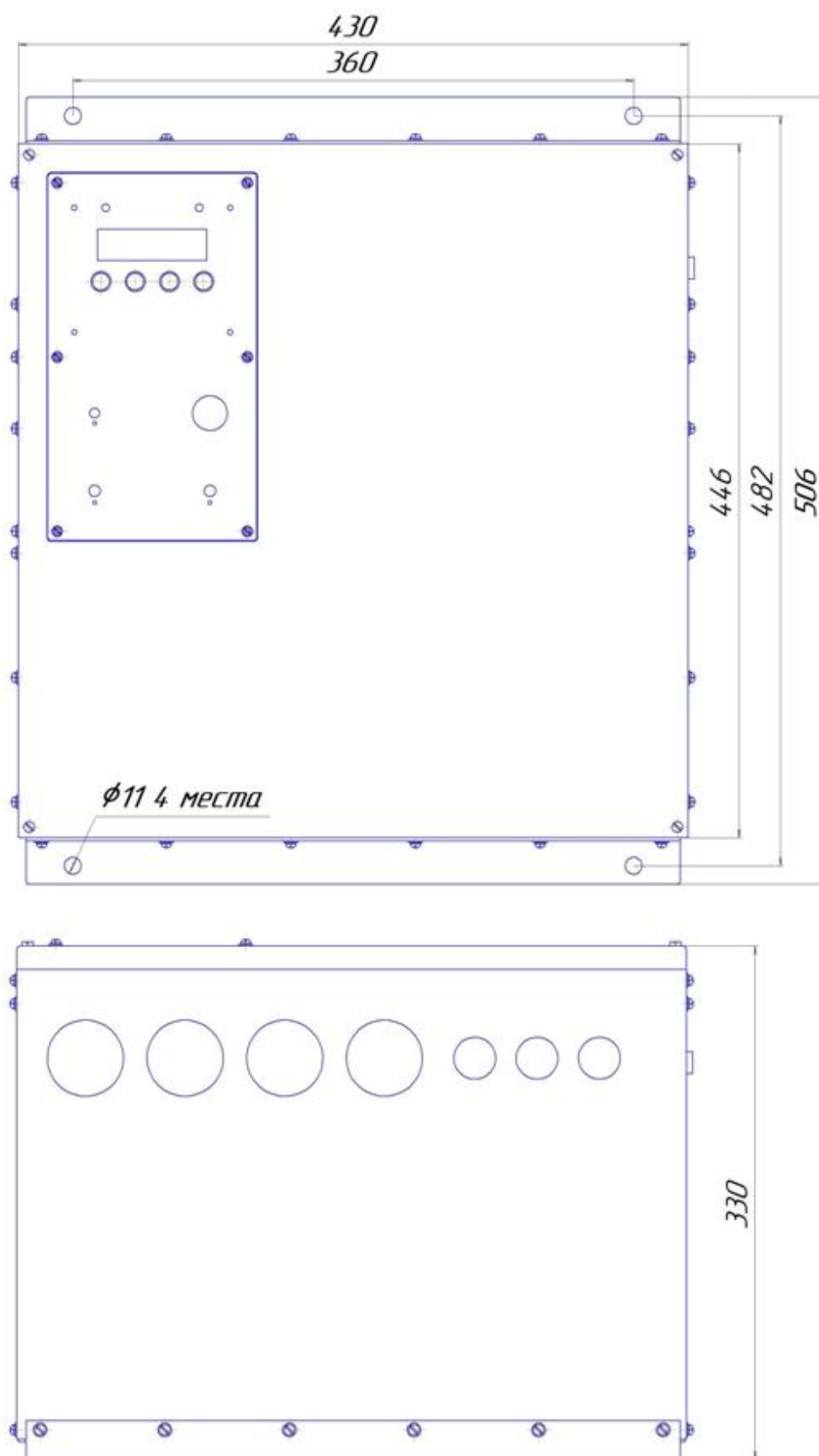
Рисунок Б6 Навесной вариант использования RBP-M-250-24, RBP-M-250-36. Крепежные уголки – сверху и снизу.
