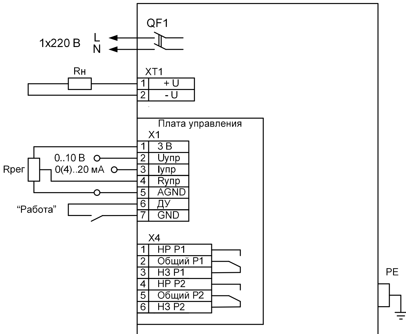
Рисунок А1 Схема подключения RBP-M-250-12, питание - однофазное
