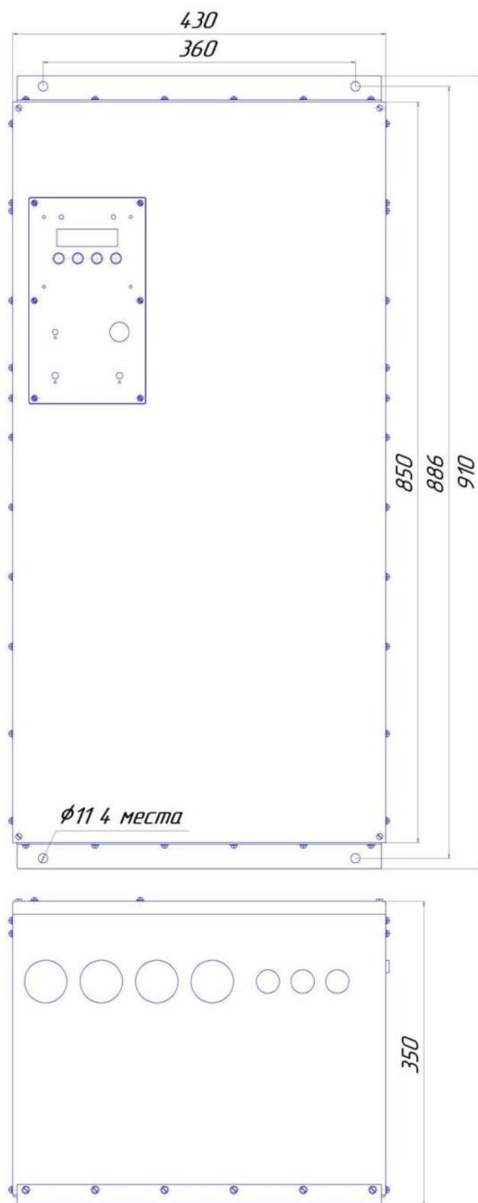
Рисунок Б9 Навесной вариант использования RBP-M-250-48, RBP-M-250-60, RBP-M-250-72. Крепежные уголки – сверху и снизу.
