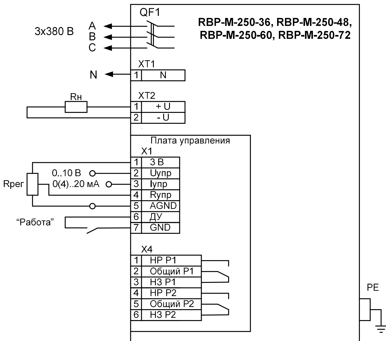
Рисунок А3 Схема подключения RBP-M-250-36, RBP-M-250-48, RBP-M-250-60, RBP-M-250-72, питание – трехфазное с нулевым проводом
